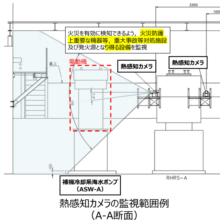
図 1 7 海水ポンプ室
