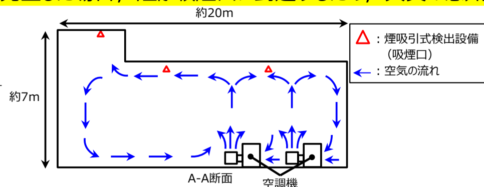
図7 主蒸気管トンネル室における空気の流れ
