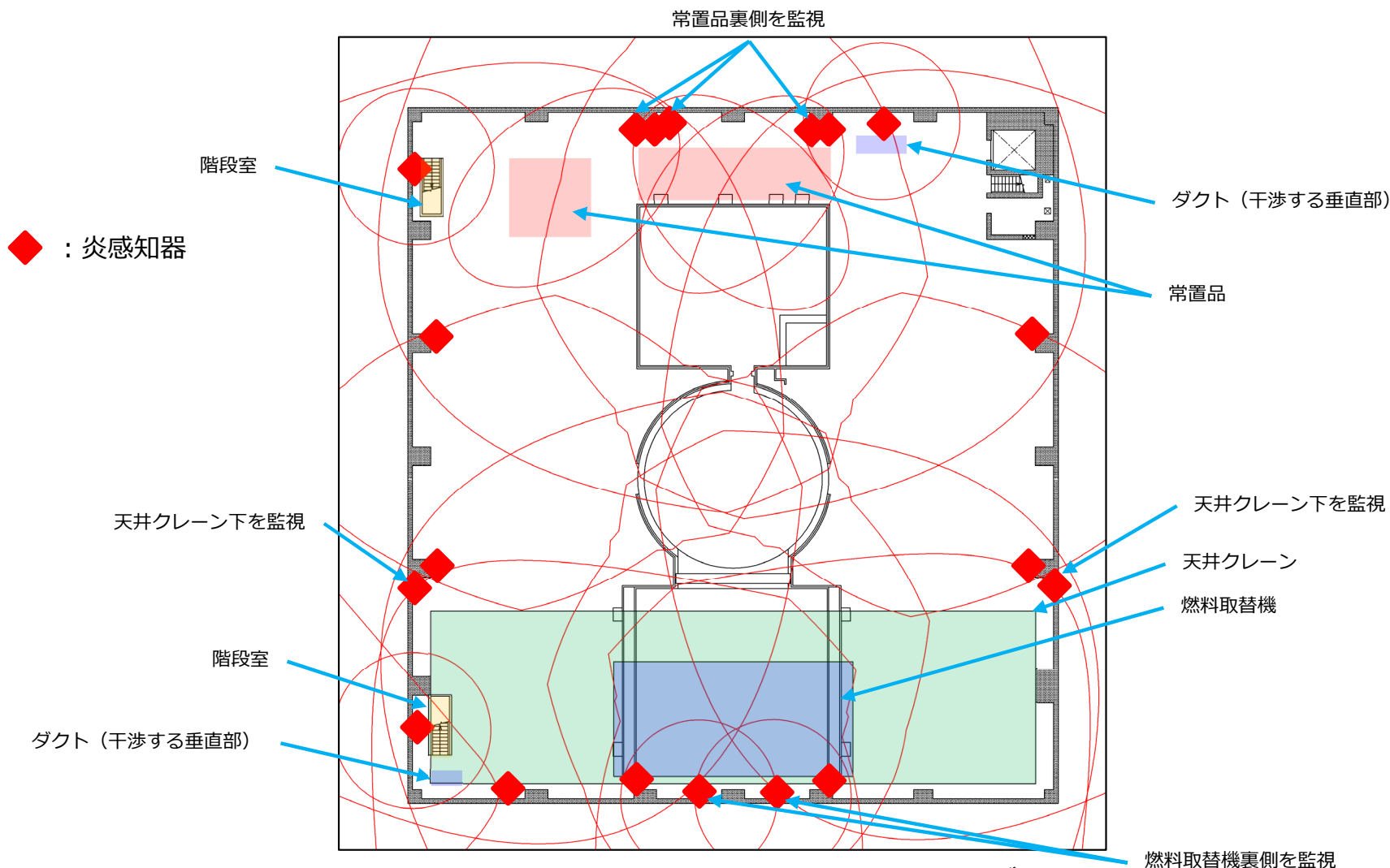
図5 原子炉建屋原子炉棟6階（オペレーティングフロア）
