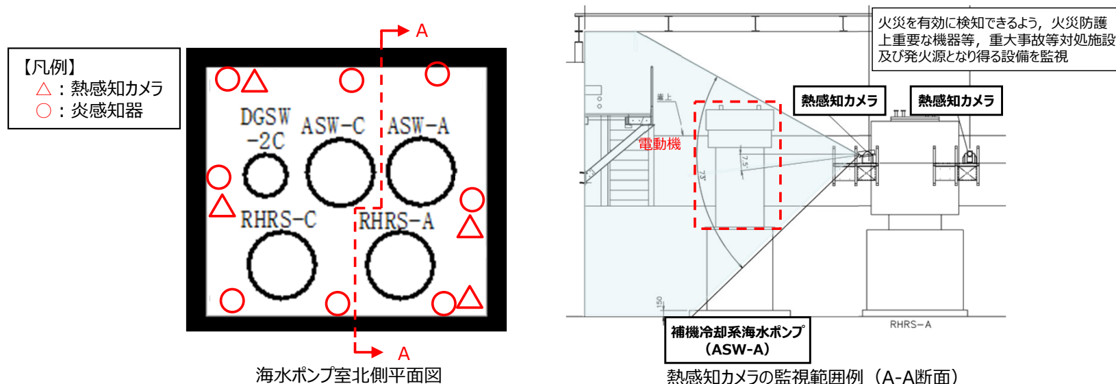
図5-1 屋外開放の火災区域・火災区画の監視範囲例（海水ポンプ室）
