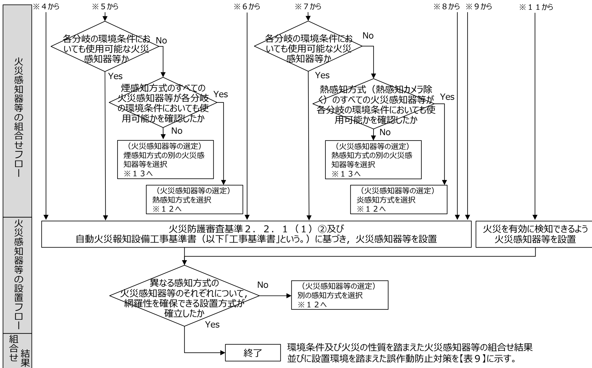
図 1 火災感知器等の選定、組合せ及び設置の設計フロー (6 / 6)
