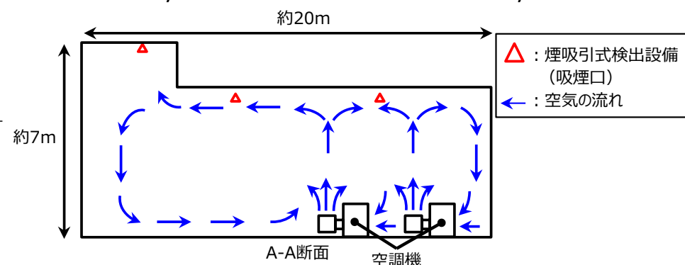
図7-2 主蒸気管トンネル室における空気の流れ
