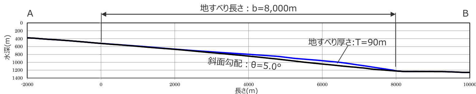
s5地点の海底地すべり断面図
