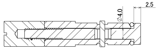
断面図 B-B
