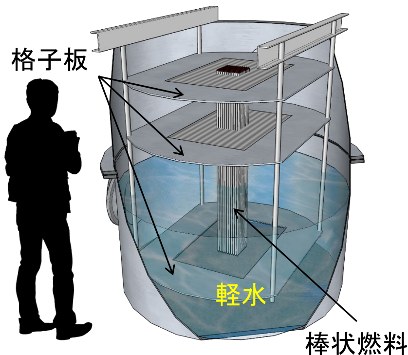
炉心タンク (直径 約180cm、高さ 約190cm)
