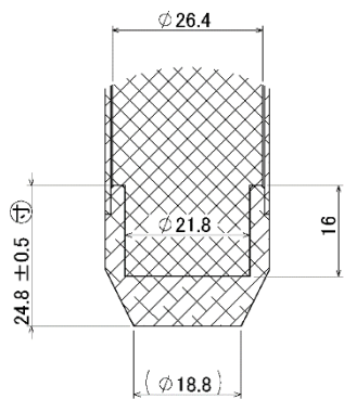
詳細図 C
