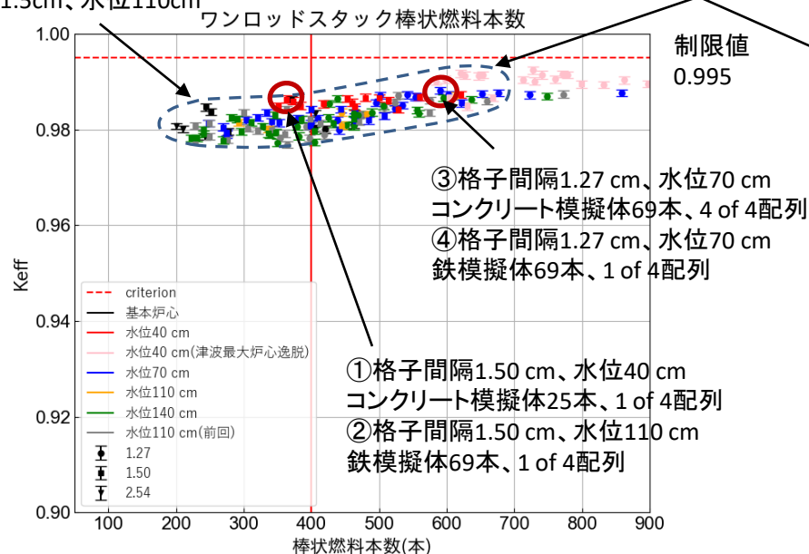
(a)ワンロードスタックマージンの評価結果
