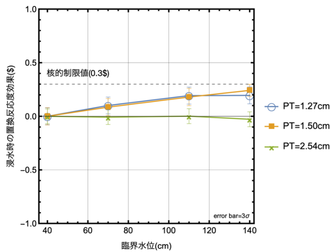
図付 2-2 内挿管（太径内挿管 3 本）の浸水による置換反応度の計算結果
