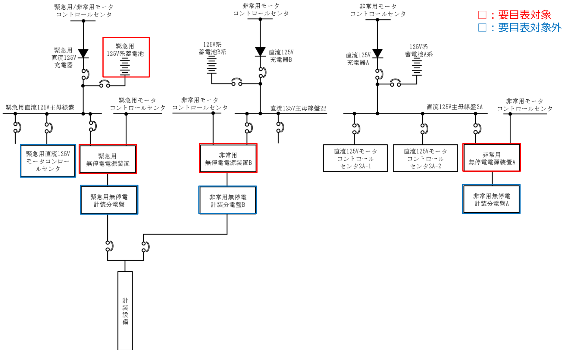
参考1図1 単線結線図
