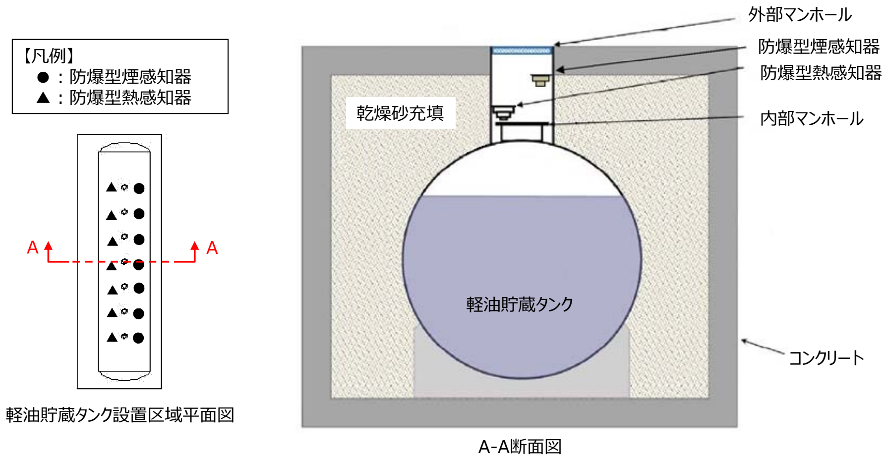
図10 軽油貯蔵タンク設置区域
