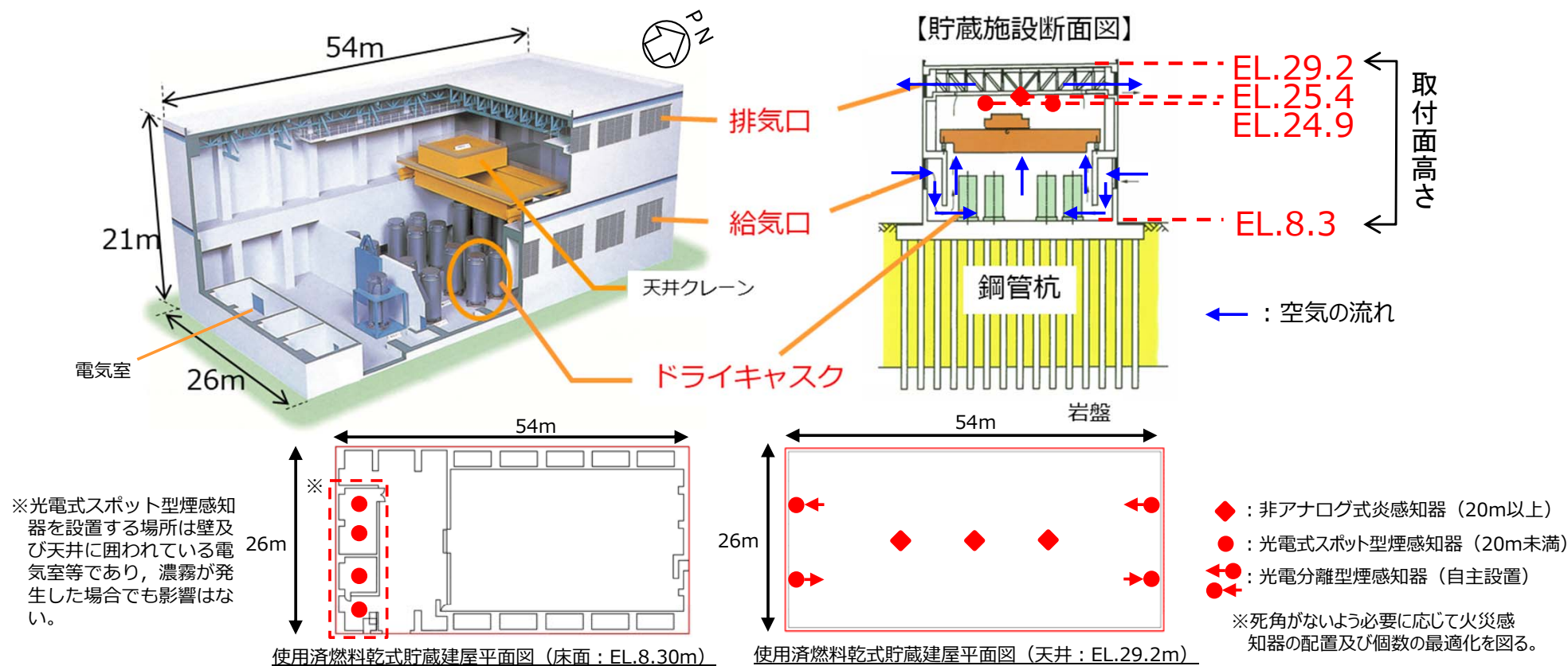
図8 使用済燃料乾式貯蔵建屋
