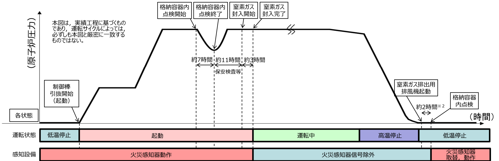
図3 原子炉の状態における原子炉格納容器内の感知
