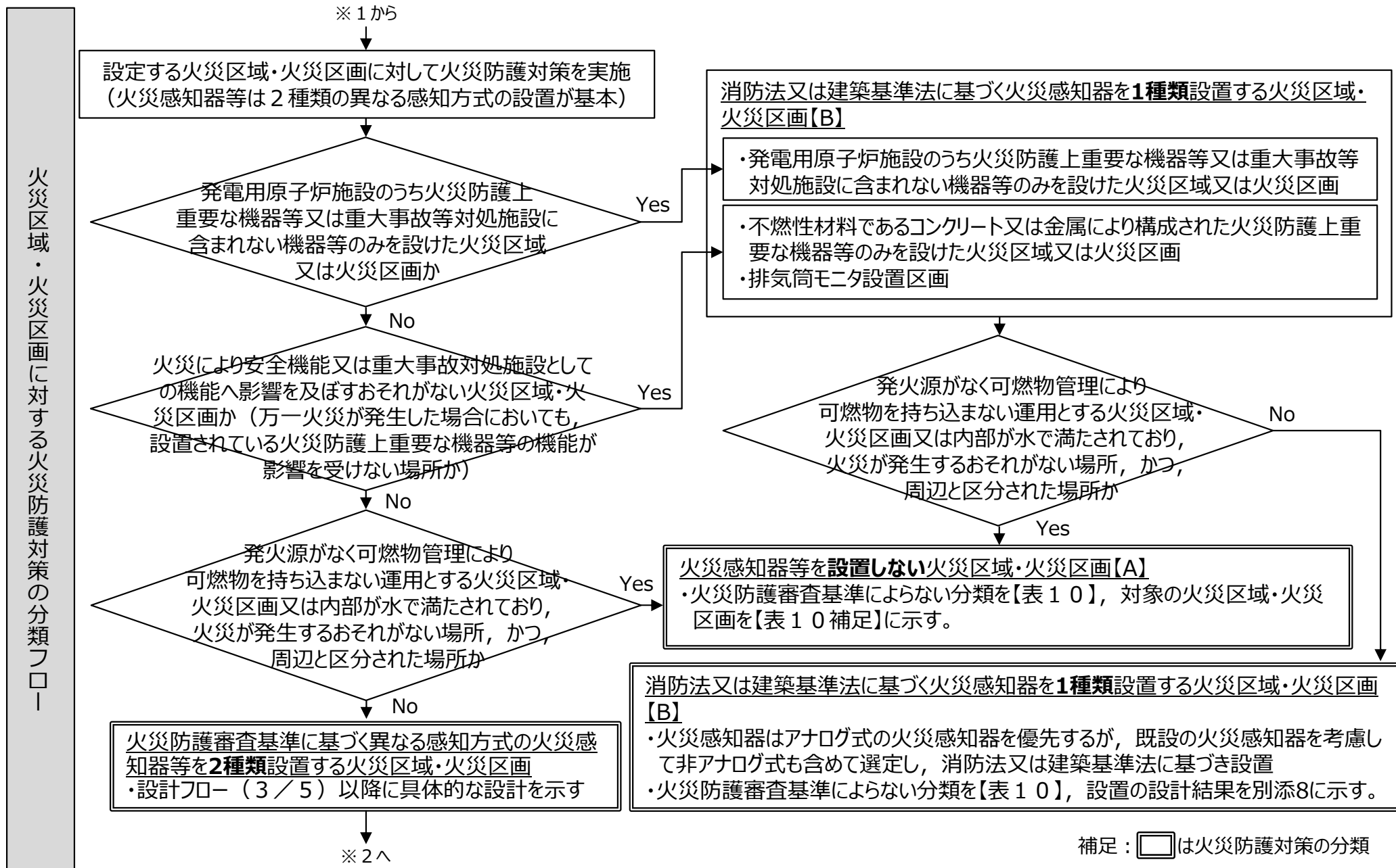
図 1 火災感知器等の選定、組合せ及び設置の設計フロー (2 / 6)
