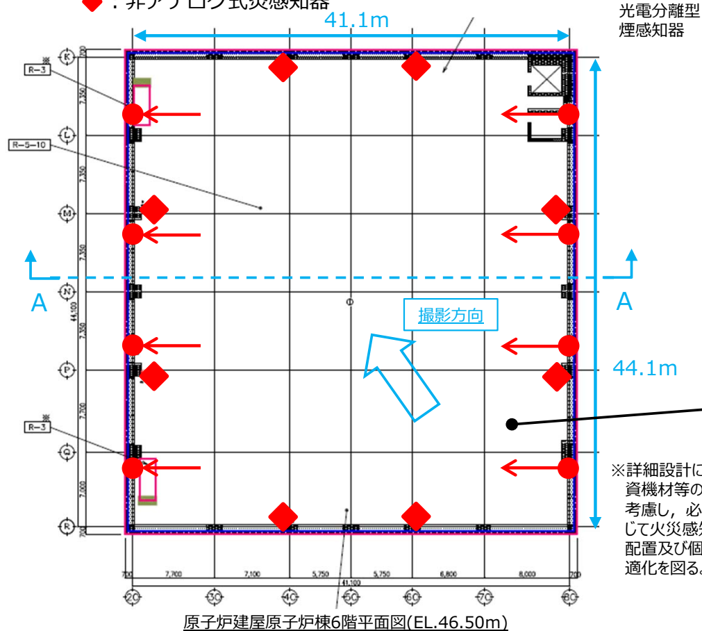
図4 原子炉建屋原子炉棟6階（オペレーティングフロア）
