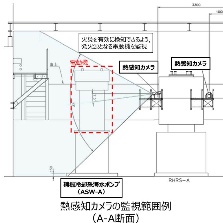
図9 海水ポンプ室
