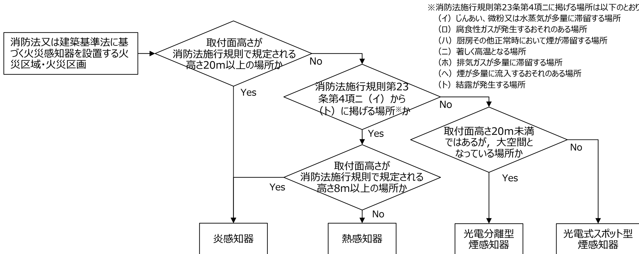
図7 消防法又は建築基準法に基づき火災感知器を1種類選択する火災区域・火災区画の火災感知器の選択フロー
