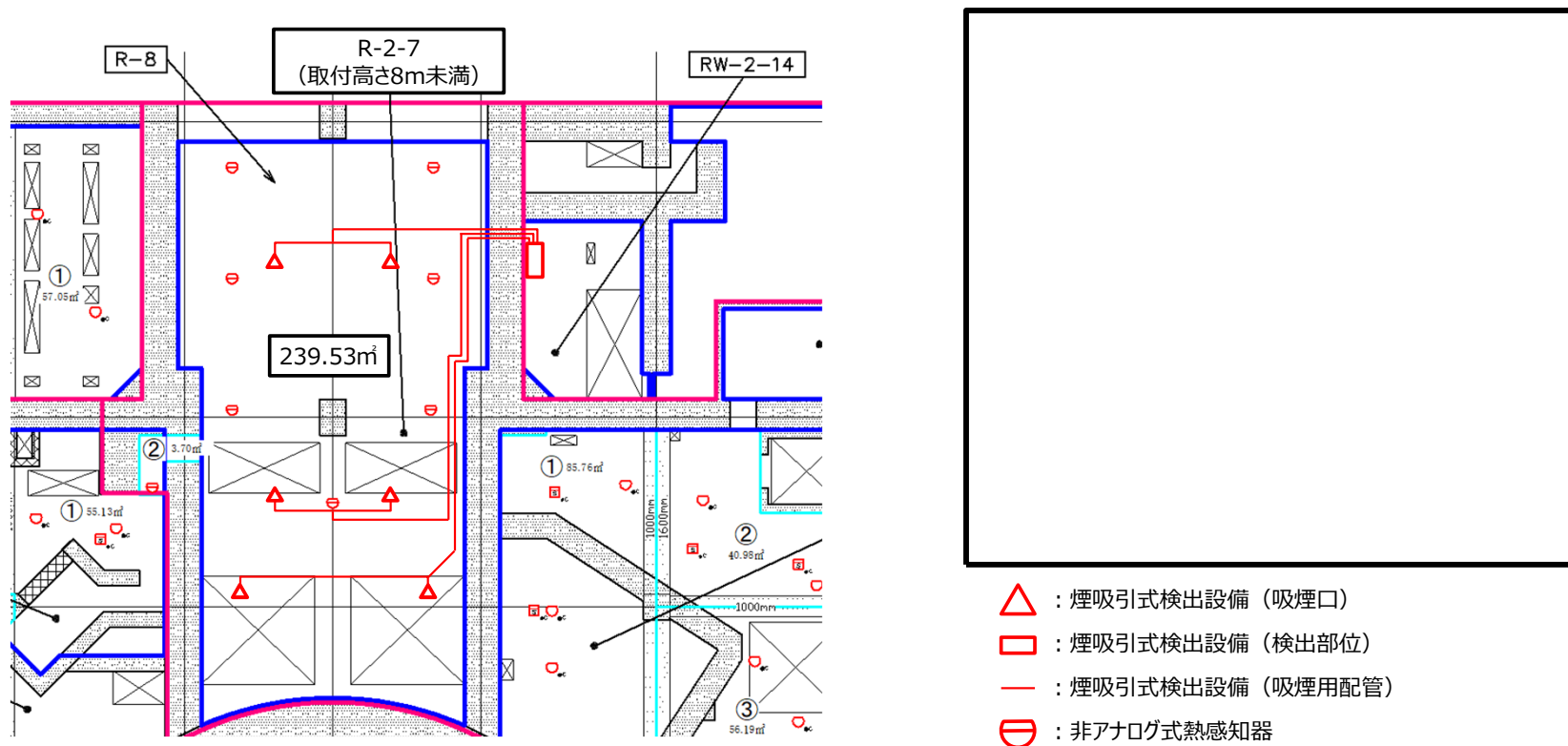
図5 主蒸気管トンネル室
