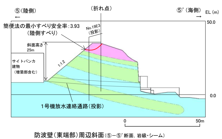
図5 グループAの地質断面図
