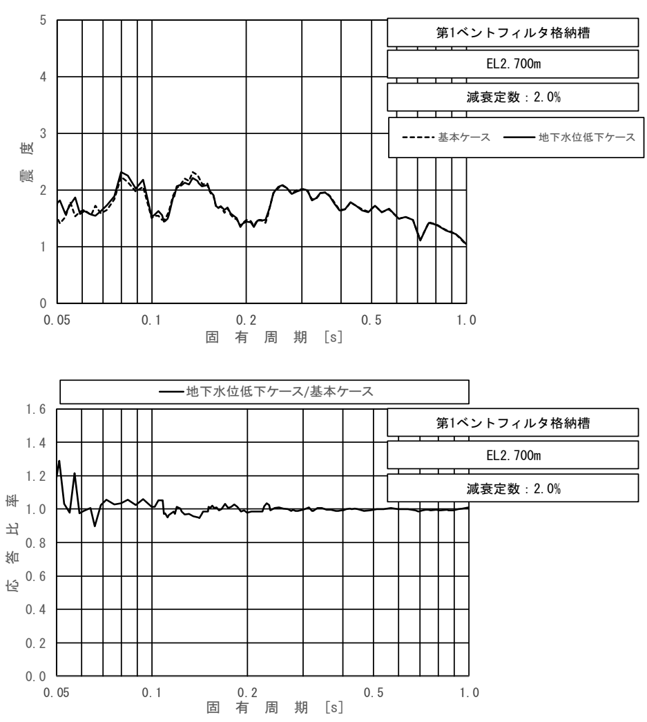
図 3.1.6-1 (3/3) 床応答スペクトル (第1ベントフィルタ格納槽) (基準地震動 S_s - D (++) , 水平方向 (NS), EL. 700m, 減衰 2.0%)
