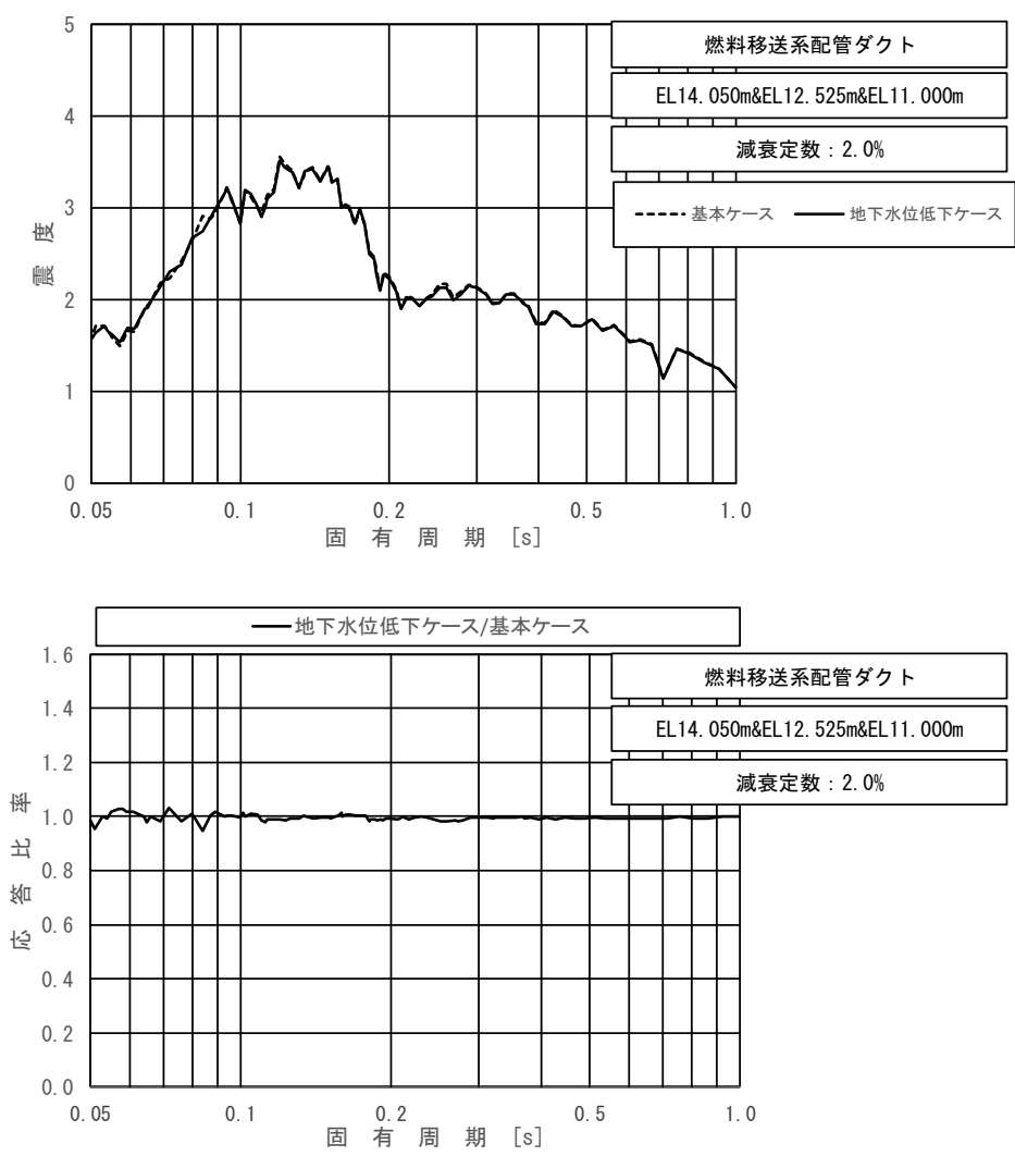
図 3.1.4-5 床応答スペクトル (屋外配管ダクト (B-ディーゼル燃料貯蔵タンク～原子炉建物) (燃料移送系配管ダクト)) (基準地震動 S s -D (++) , 水平方向, EL14.050m～EL11.000m, 減衰 2.0%)
