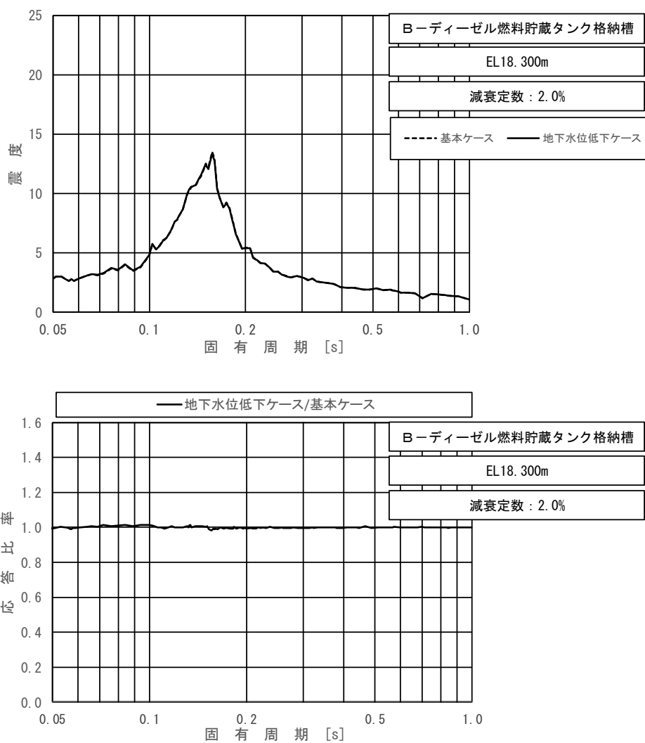
図 3.1.3-1 (1/5) 床応答スペクトル (B-ディーゼル燃料貯蔵タンク格納槽) (基準地震動 S s - D (++) , 水平方向 (N S) , EL18.300m , 減衰 2.0%)
