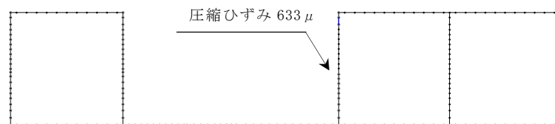
図 3-20 曲げ・軸力系の破壊に対する照査におけるひずみの時刻歴波形 (解析ケース①, S s -D (++) )
