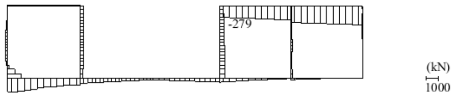
数値：評価位置における断面力 (b) 軸力 (kN) (+：引張，-：圧縮)
