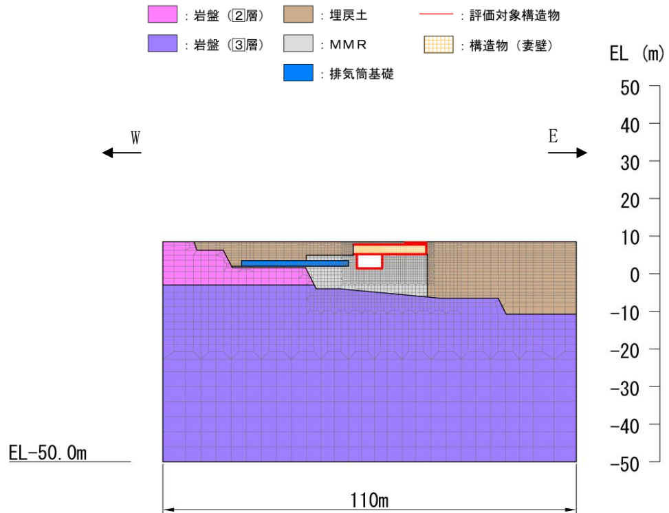
図 3-7 屋外配管ダクト (タービン建物～排気筒) 地震応答解析モデル図 (C-C 断面)
