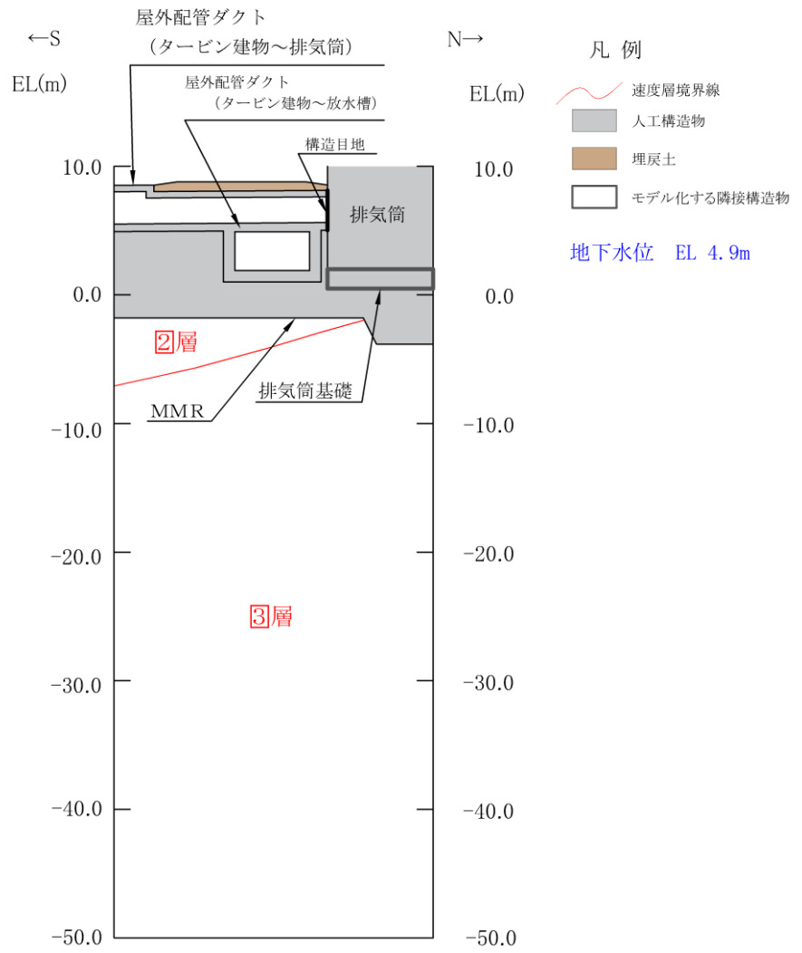
図 3-4 屋外配管ダクト (タービン建物～放水槽) との一体化部 地震時荷重算出断面図 (C-C 断面)
