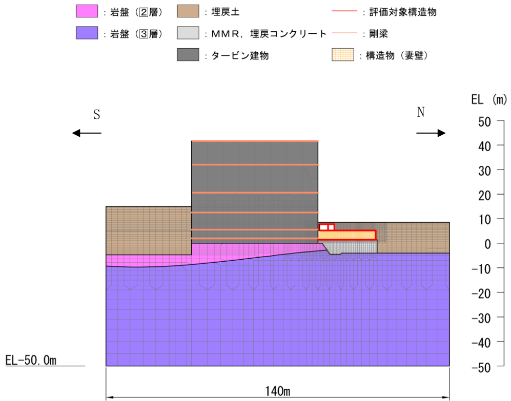
図 3-6 屋外配管ダクト (タービン建物～排気筒) 地震応答解析モデル図 (B-B 断面)
