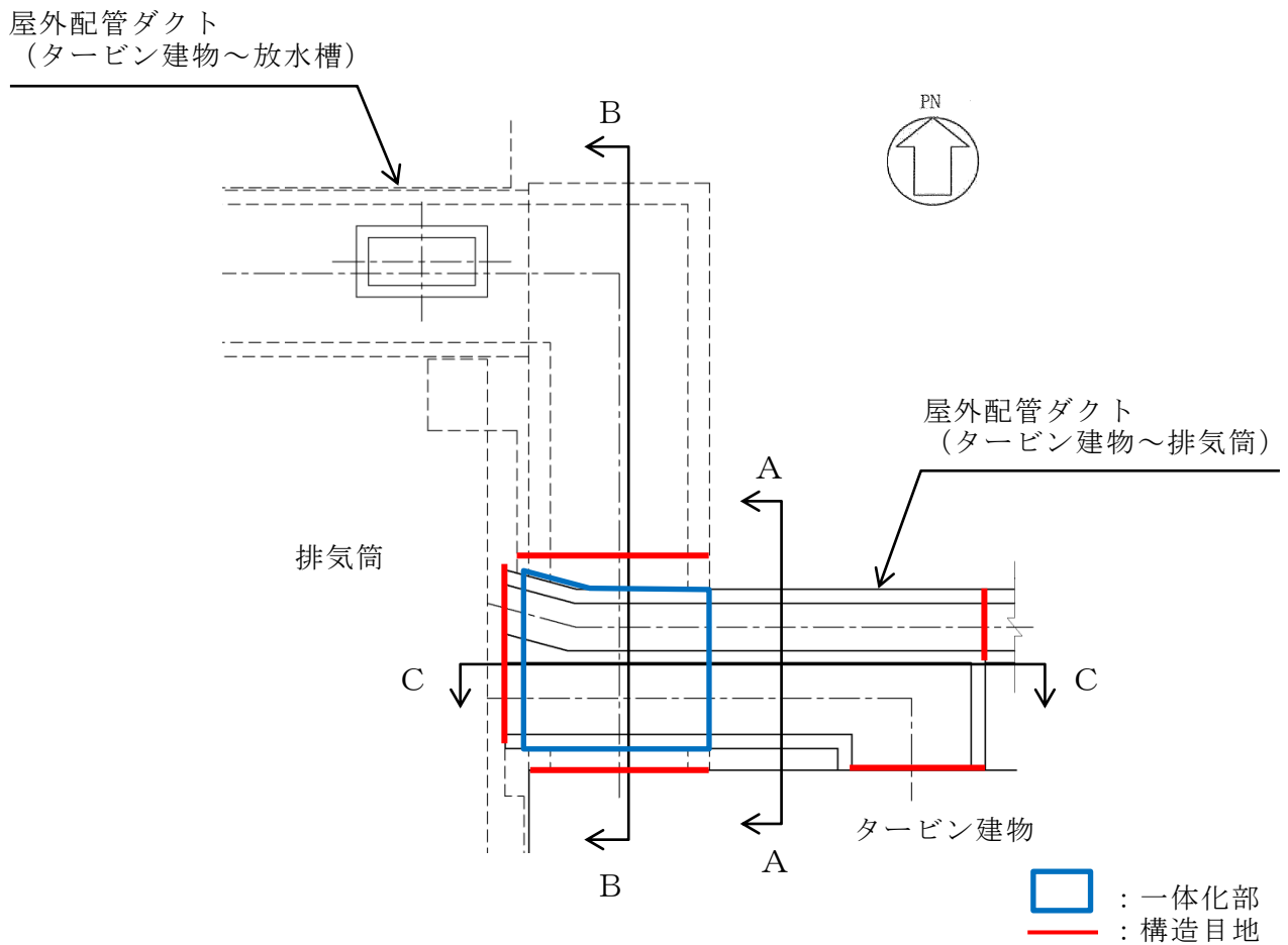
図 3-1 屋外配管ダクト（タービン建物～放水槽）との一体化部 地震時荷重算出断面位置図
