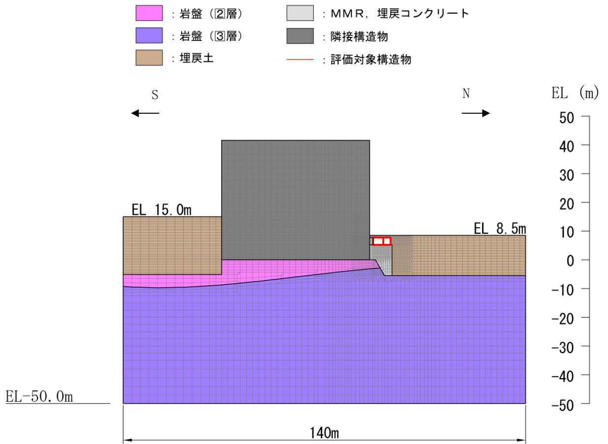
図 3-41 屋外配管ダクト (タービン建物～排気筒) 地震応答解析モデル図 (A-A 断面)
