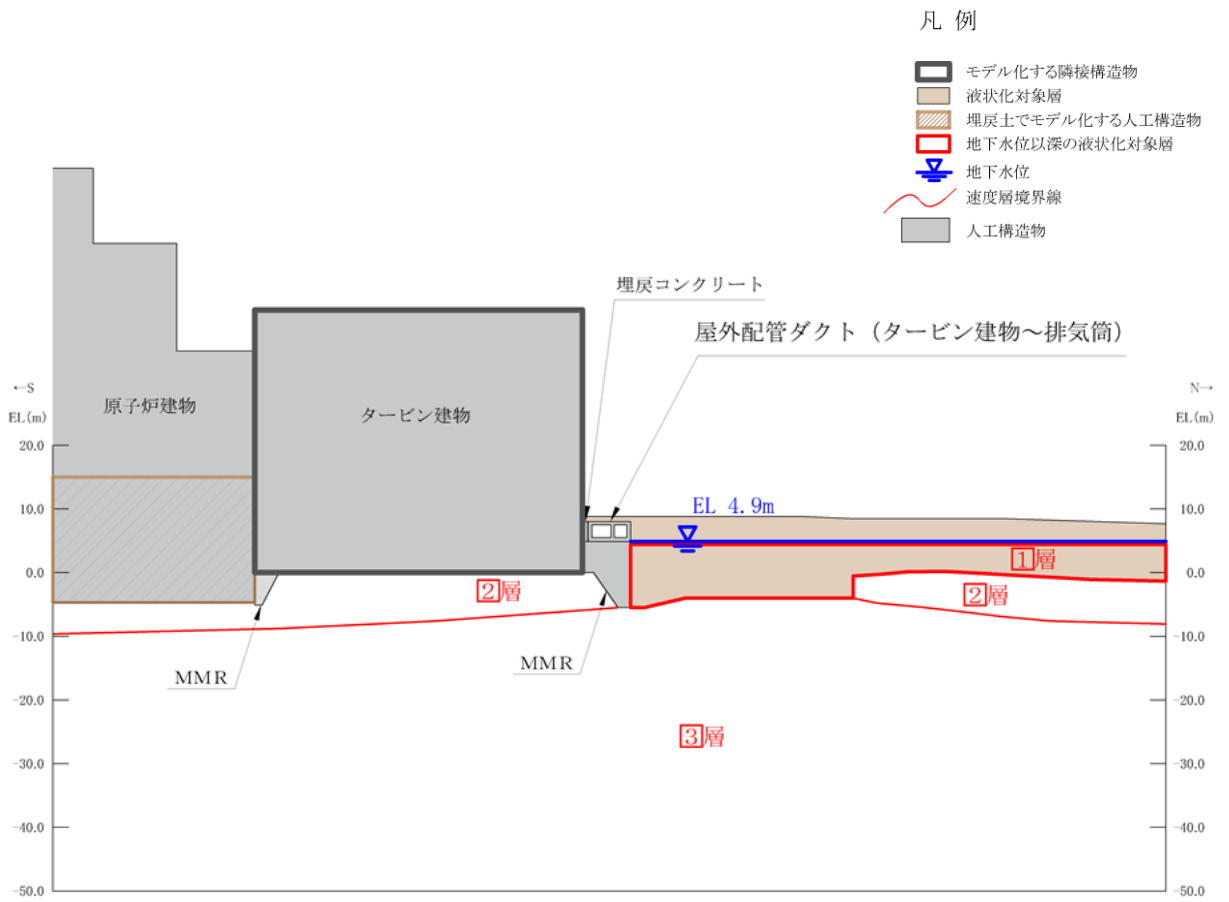
図 3-2 屋外配管ダクト (タービン建物～排気筒)
