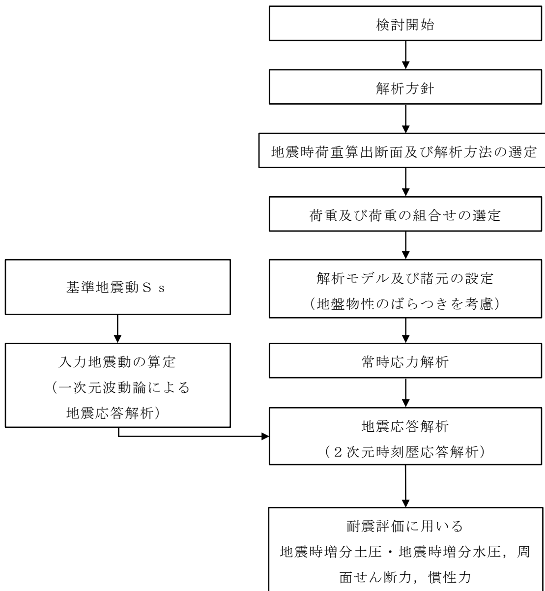
図 2-5 屋外配管ダクト (タービン建物～排気筒) の地震応答解析フロー
