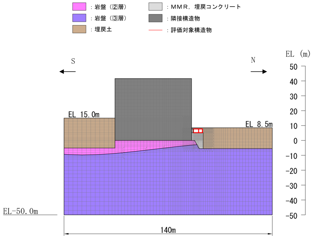
図 3-5 屋外配管ダクト (タービン建物～排気筒) 地震応答解析モデル図 (A-A 断面)
