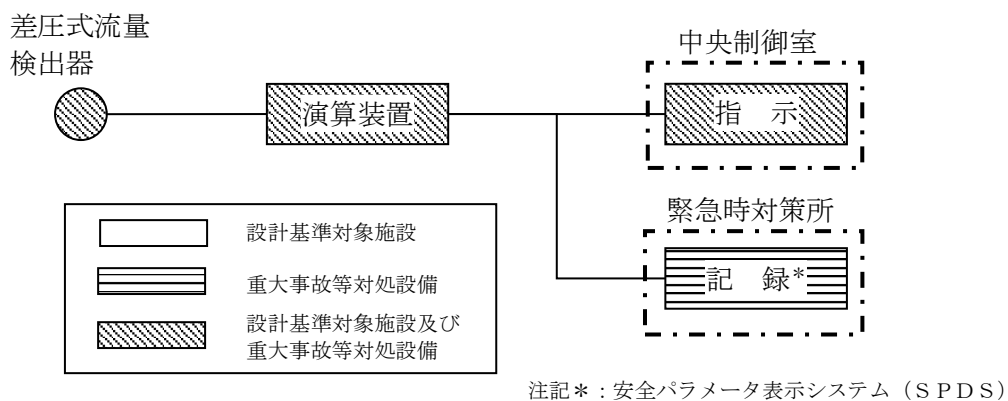
図 3-94 残留熱除去系熱交換器冷却水流量の概略構成図
