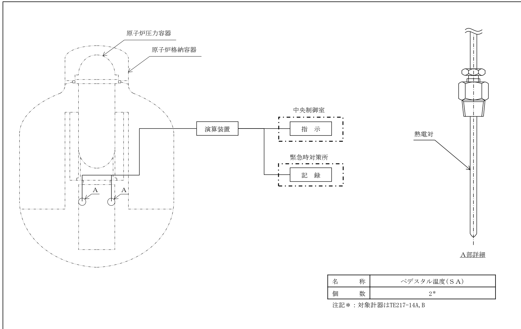
図 3-50 検出器の構造図 (ペDESTAL温度 (S A))
