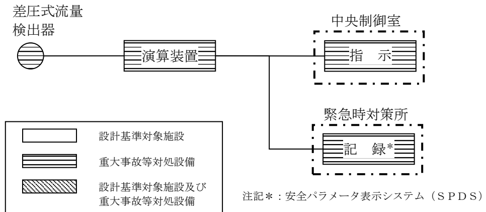
図3-67 格納容器代替スプレイ流量の概略構成図
