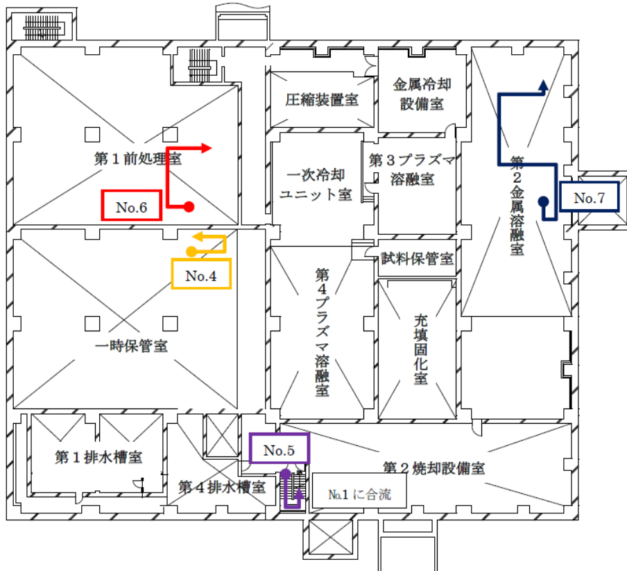
減容処理棟建家平面図（地下中1階）
