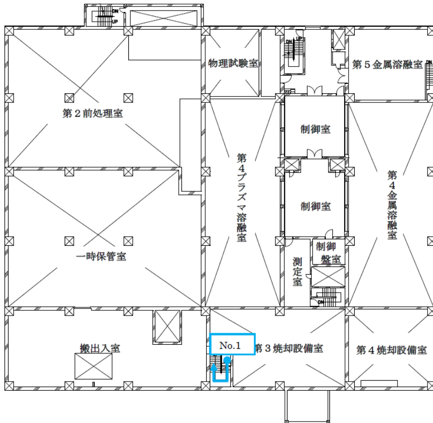
減容処理棟建家平面図（中2階）
