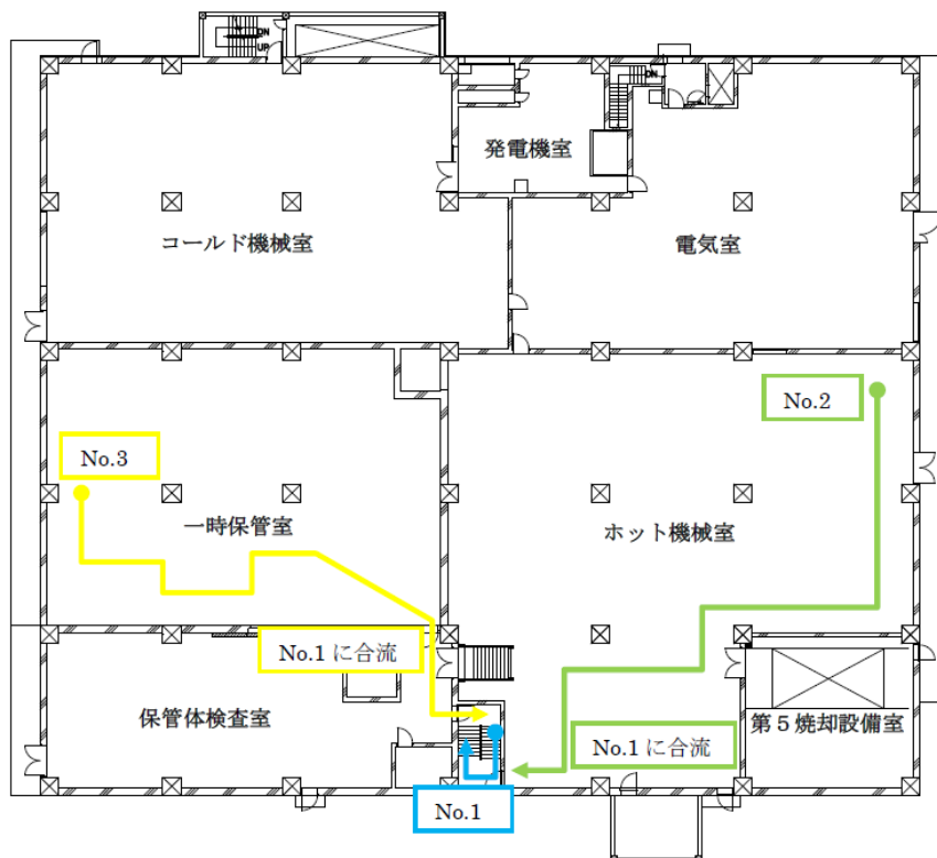
減容処理棟建家平面図（2階）
