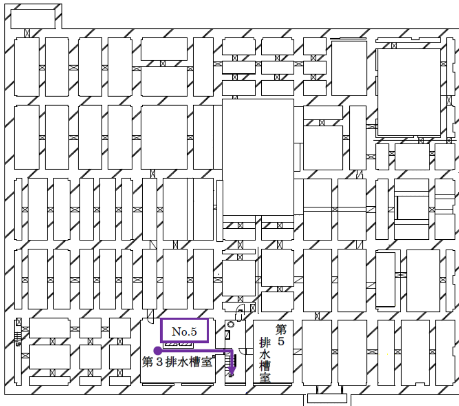
減容処理棟建家平面図（基礎スラブ階）
