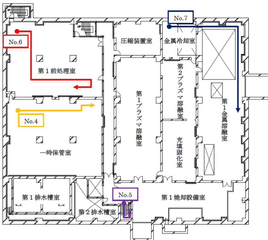
減容処理棟建家平面図（地階）
