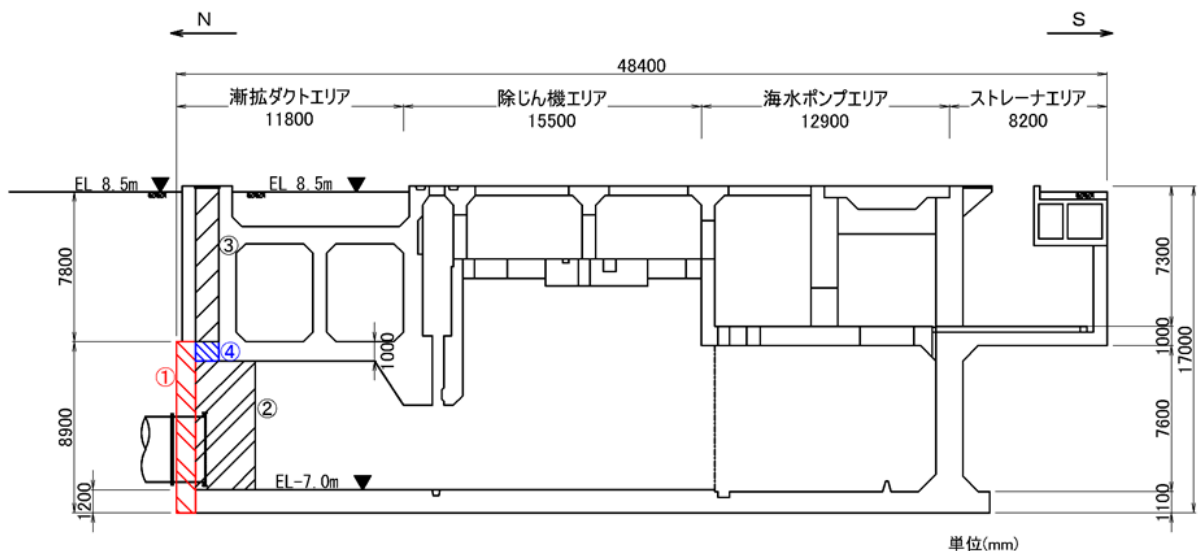
図2-6 補強工事实施部材位置
