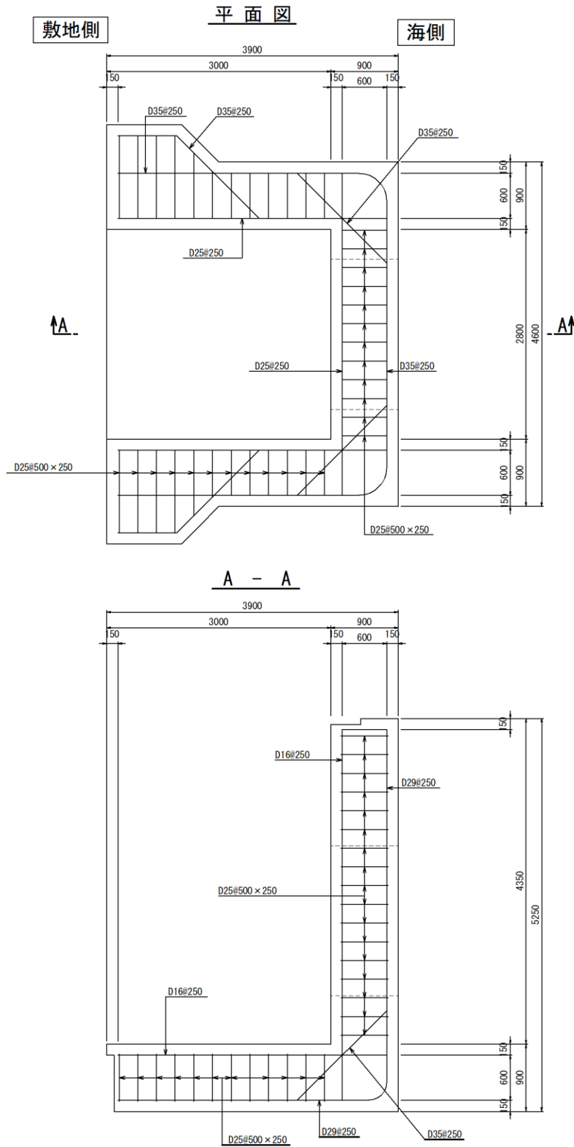
图 9-1(1) 概略配筋图 (集水榭 (屋外排水路逆止弁①))
