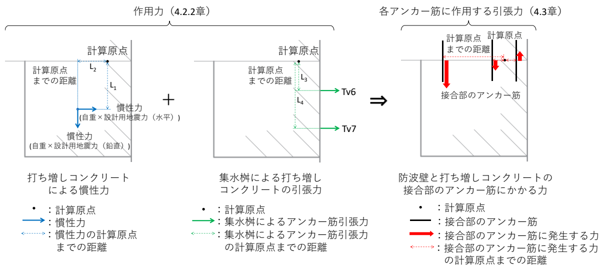
図4-4(1) 作用力の計算概要 (屋外排水路逆止弁⑦のイメージ)
