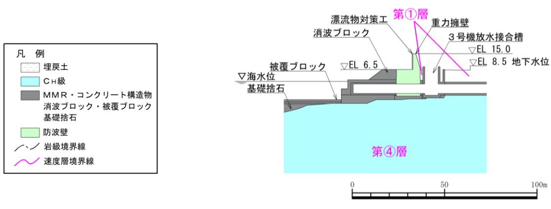
図 5-3(3) 地質断面図 (防波壁 (波返重力擁壁) ③-③断面 (参考))
