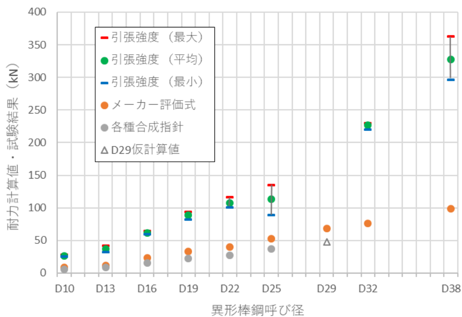
図 4-3 (1) 評価式による耐力と試験結果の比較 (引張, 平成 9 年度)
