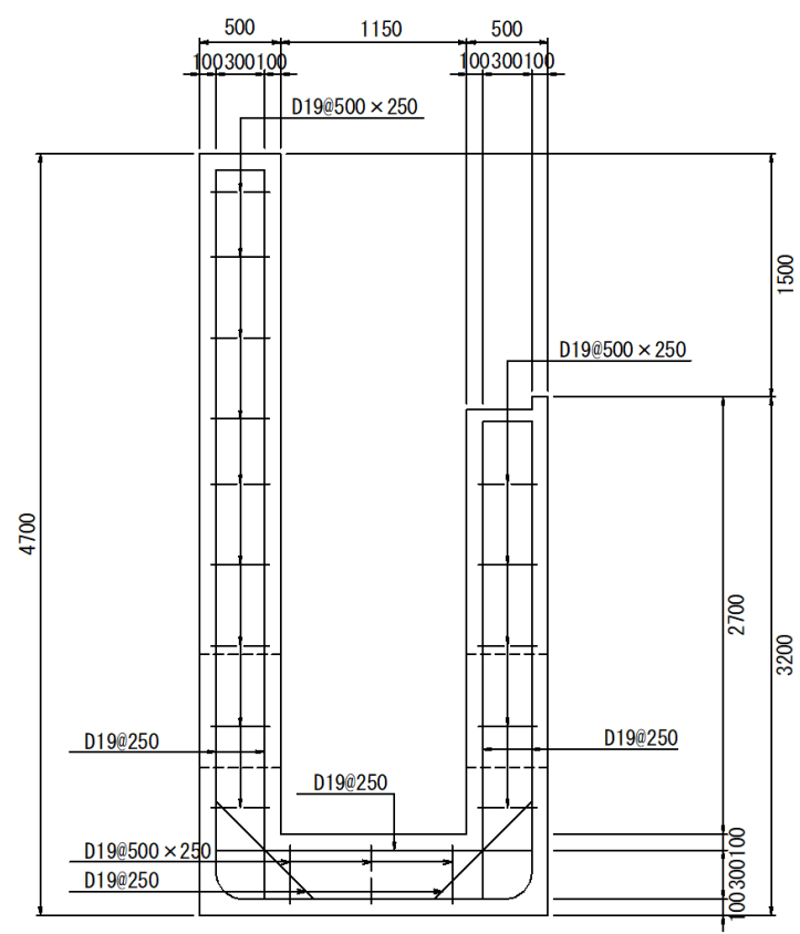
図 9-1(3) 概略配筋図 (集水桝 (屋外排水路逆止弁⑦))
