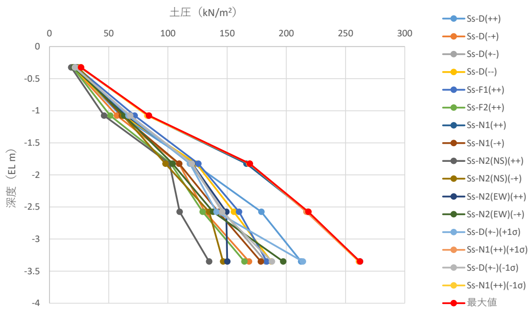
図 4-3 基準地震動 Ss の土圧分布の比較
