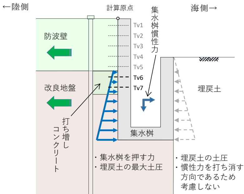
図 4-2 設計に考慮する作用荷重の考え方
