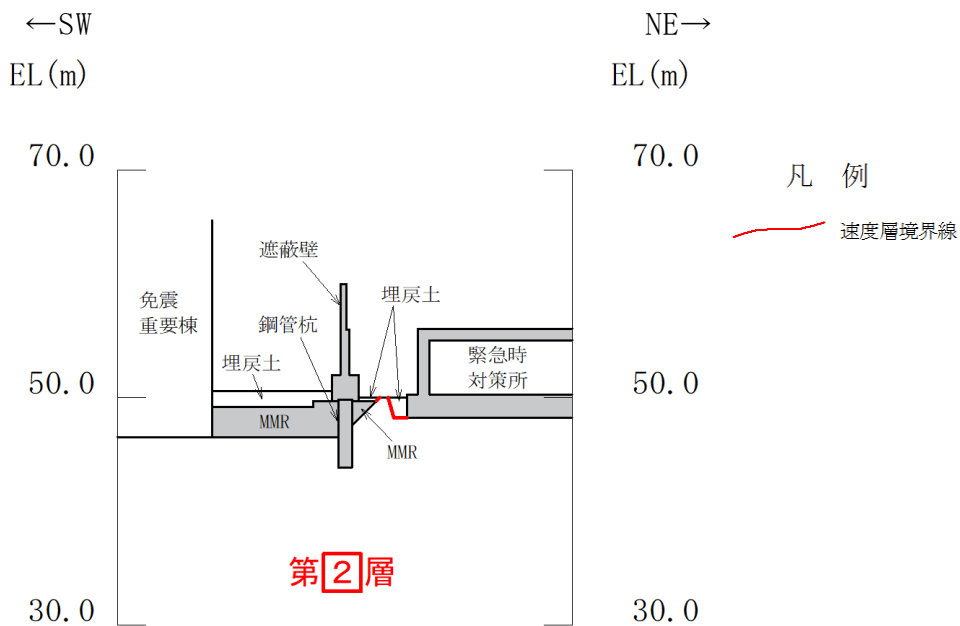
図3-2 評価対象断面図（A-A断面）
