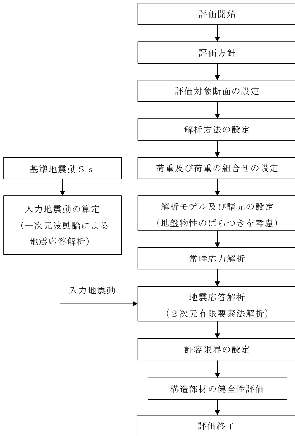
図 2-5 屋外配管ダクト（排気筒）耐震評価フロー
