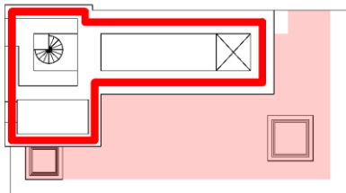
第1ベントフィルタ格納槽 EL 2700
