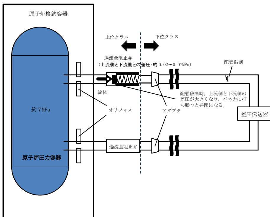
図 5-2-5 原子炉压力容器からの計装ライン構成概念図
