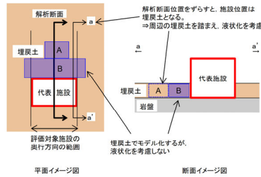
図 2.4.4-4(1) 隣接施設のモデル化の考え方
