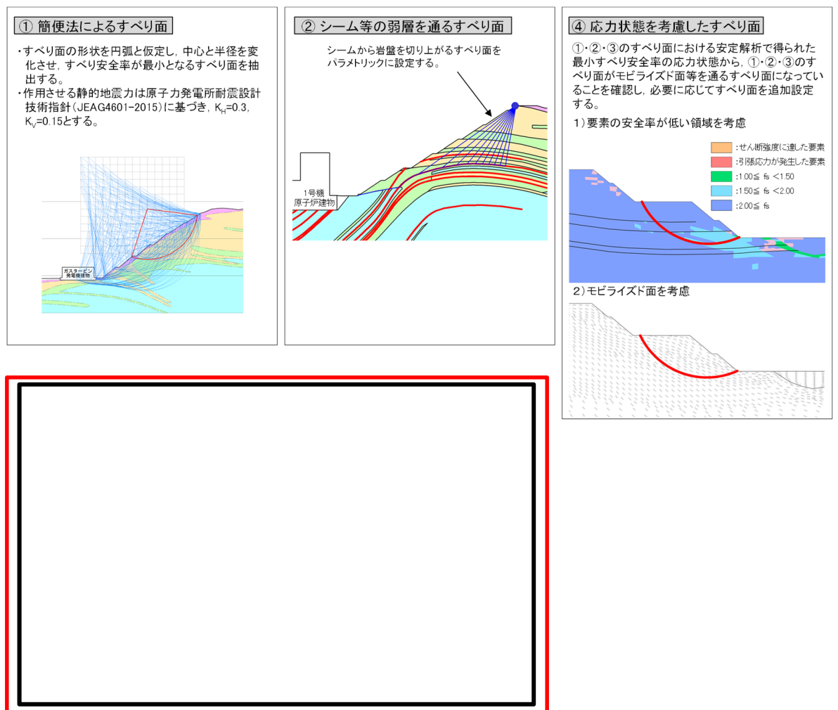
図 3.4.3-1 想定すべり面の設定方法（赤枠追加）
