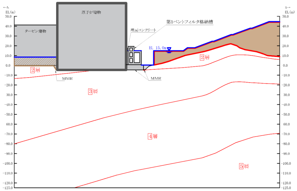
図 3-2 第 1 ベントフィルタ格納槽 評価対象断面図 (A-A 断面)
