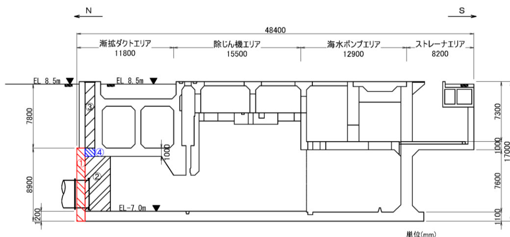
図2-8 補強工事实施部材位置
