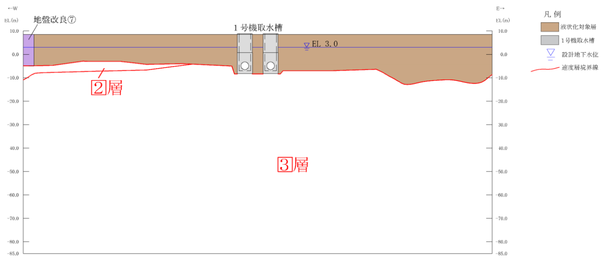
図 3-7 評価対象地質断面図 (B-B 断面)
