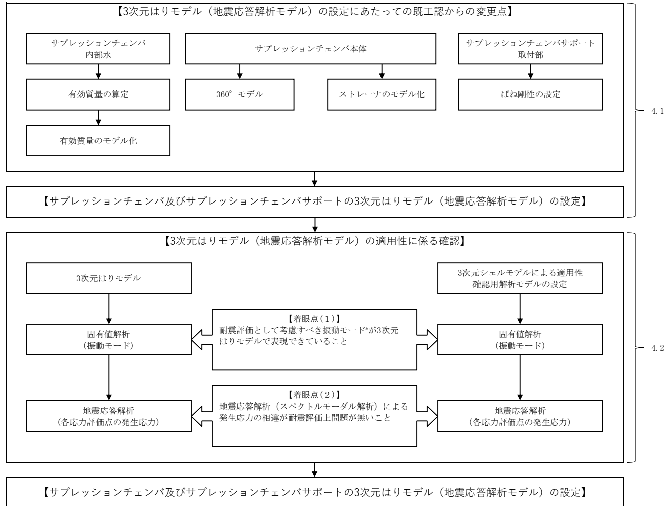
図 4.2-1 3次元はりモデル設定及び適用性検証フロー
