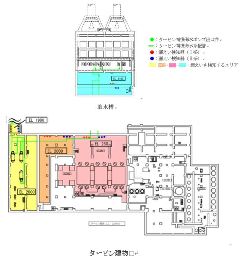
図 4-3 漏えい検知器及びタービン補機海水ポンプ出口弁配置図
