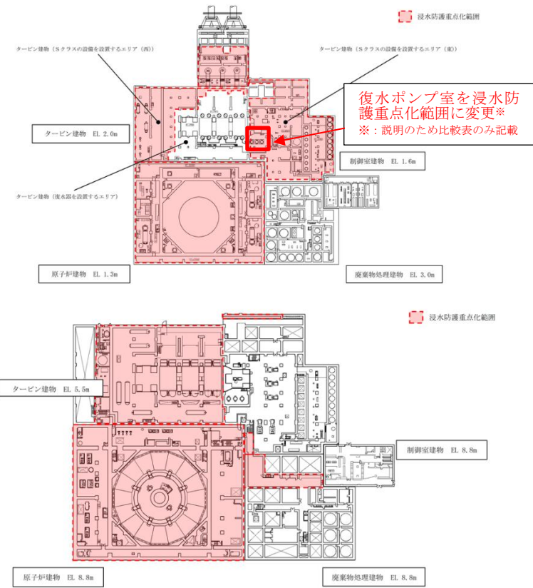
図 3-29(1) 浸水防護重点化範囲 (平面図) (1/4)
