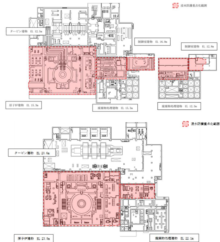
図 3-29(2) 浸水防護重点化範囲 (平面図) (2/4)
