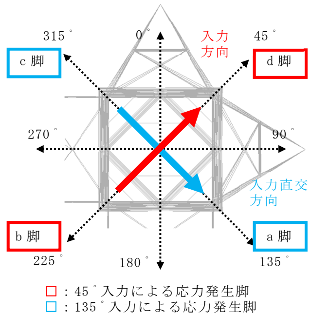
図 1.3.6-5 入力方向と主柱材発生応力の関係
