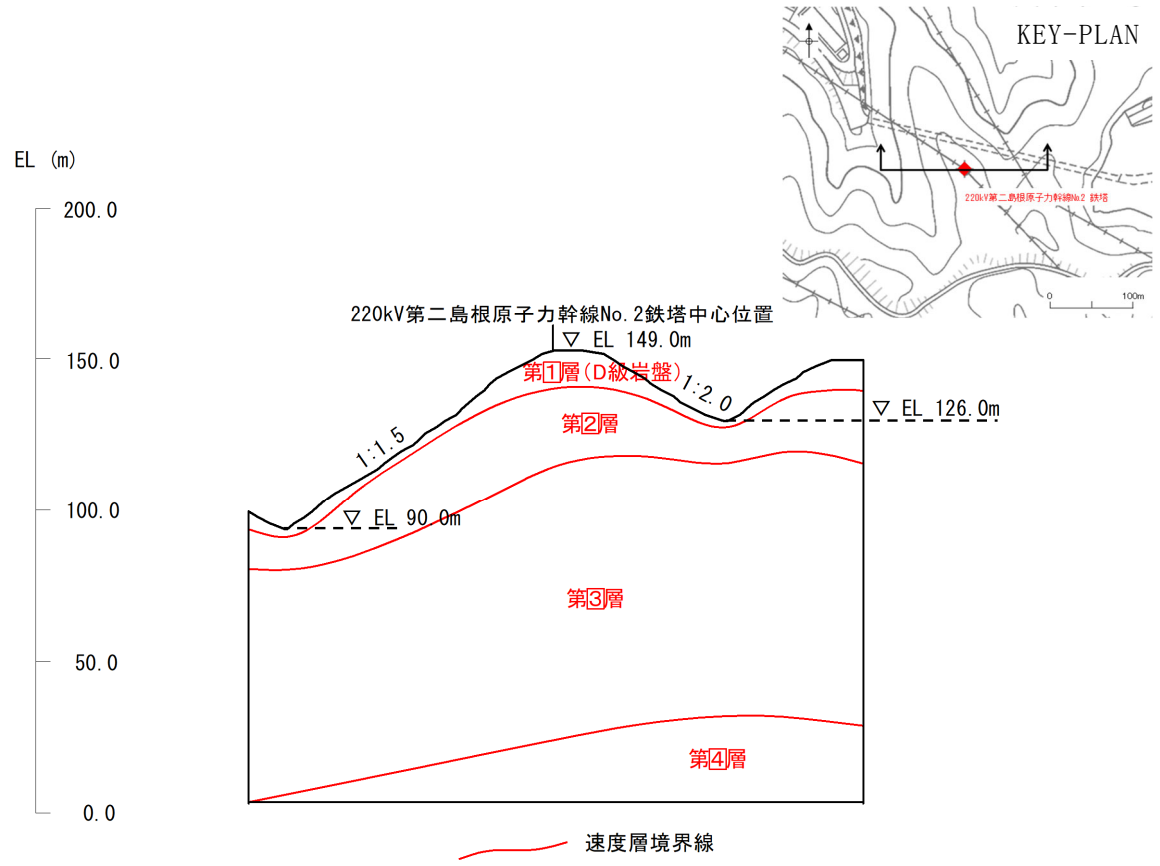
図1.1.10-22 220kV第二島根原子力幹線No.2鉄塔 地質断面図(速度層区分)
