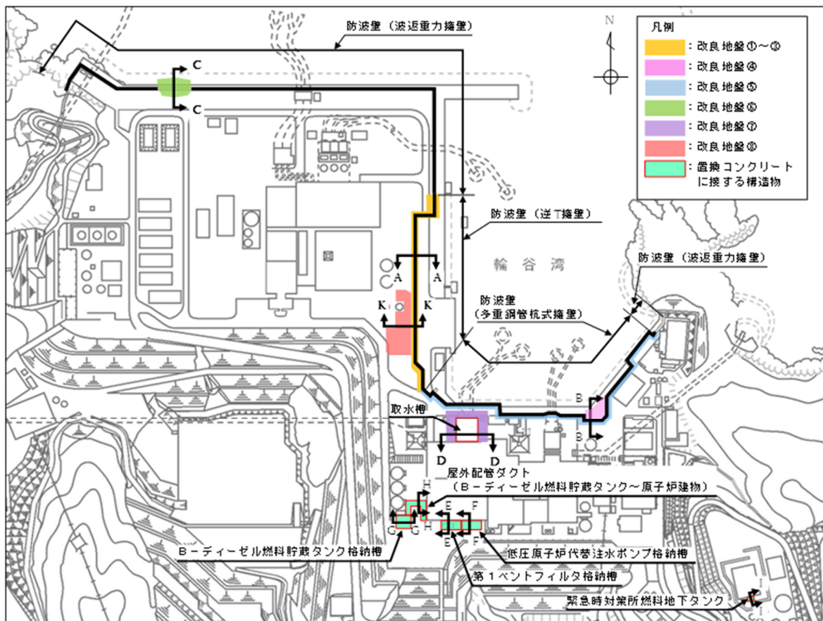
図1.1.10-14 改良地盤を設置する施設の平面配置図
