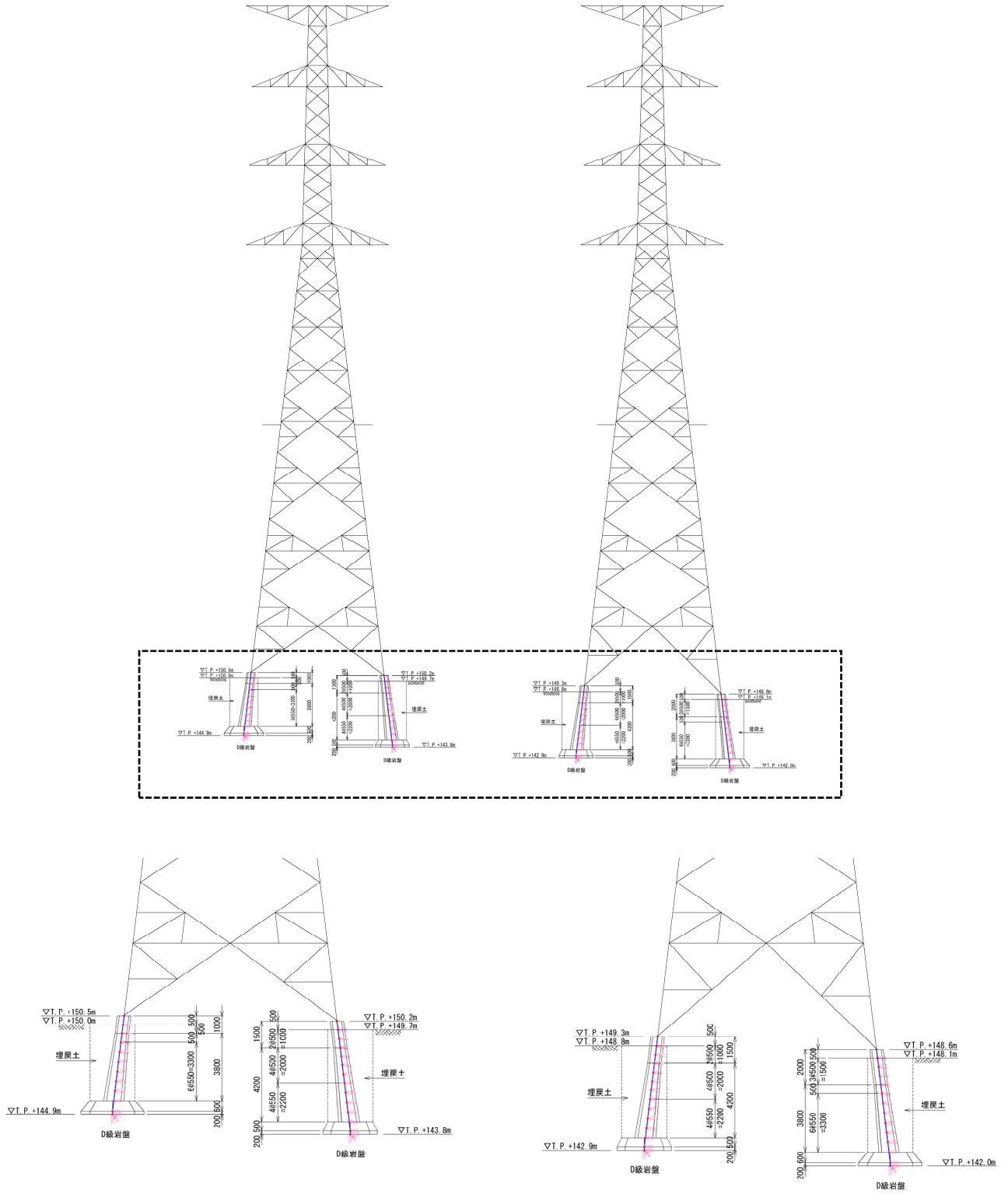
図 1.1.10-30 220kV 第二島根原子力幹線 No.2 鉄塔基礎解析モデル
