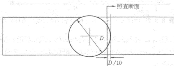
図 1.2.10-16 床板部の照査断面
