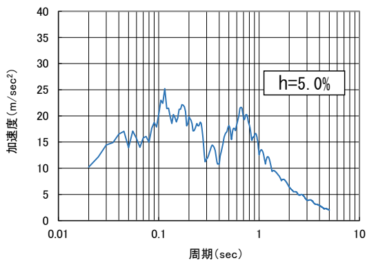
水平成分の加速度応答スペクトル
