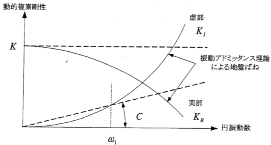
図 1.3.10-20 振動アドミタンス理論による地盤ばね
