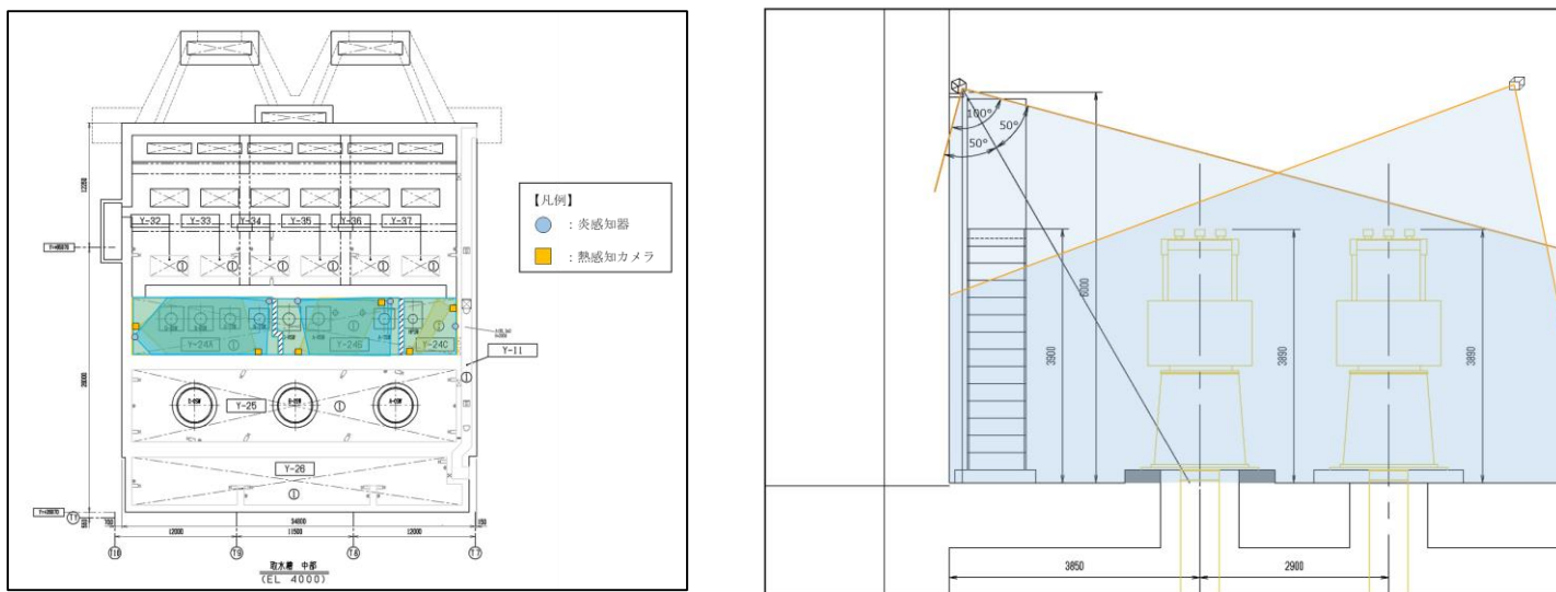
図2 海水ポンプエリアの火災感知器配置
