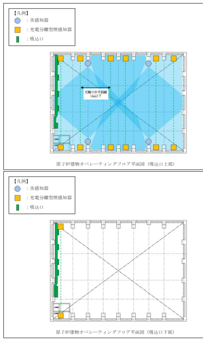
図3 原子炉建物オペレーティングフロアの火災感知器配置
