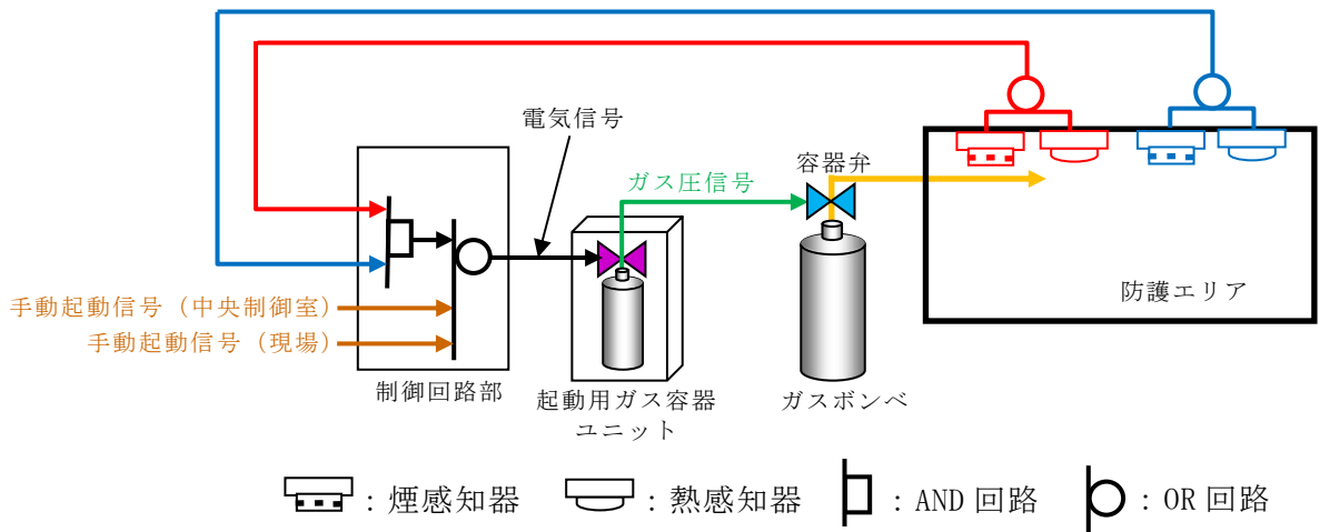
図5-1 全域ガス消火設備作動概要図
