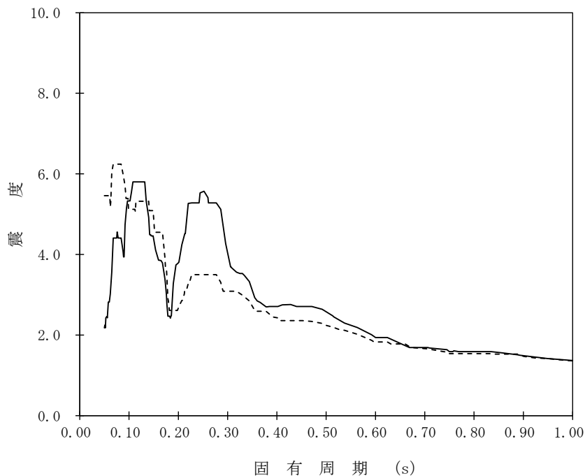
図 2-1 設計用床応答スペクトルの比較 (1/3)
