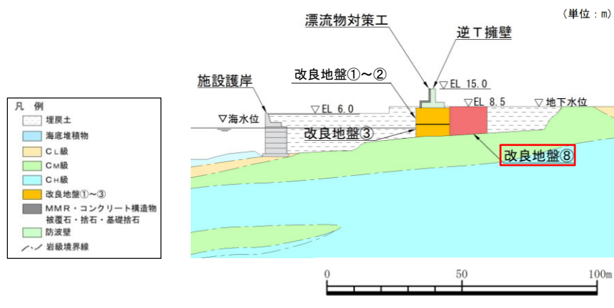
図 4.8-2 改良地盤⑧の配置図
