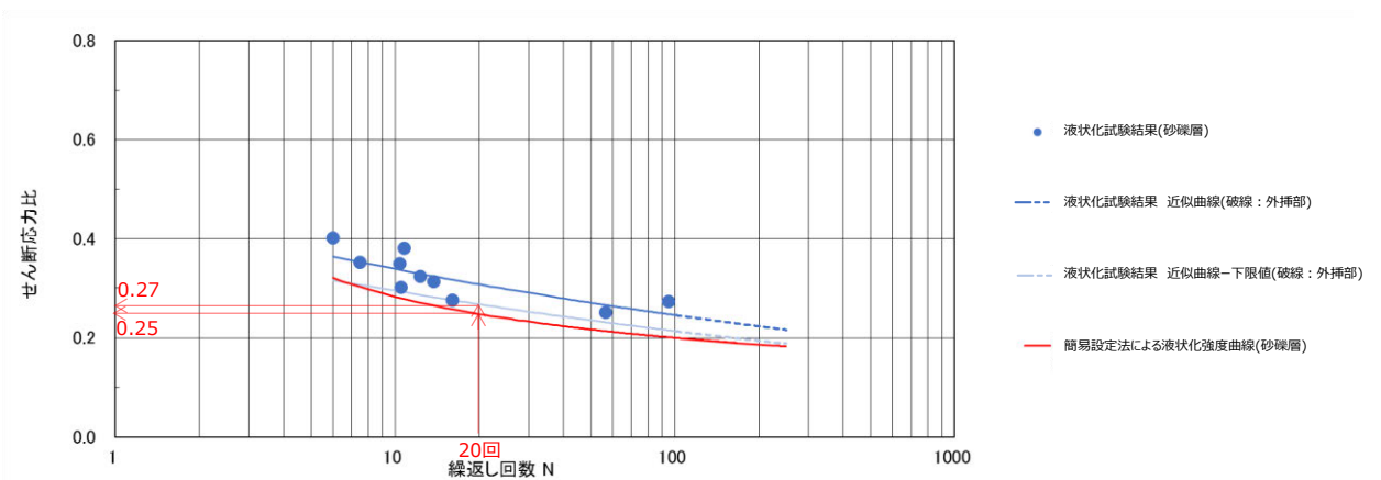
図 2-2 簡易設定法及び液状化強度試験結果による液状化強度曲線の比較（砂礫層）
