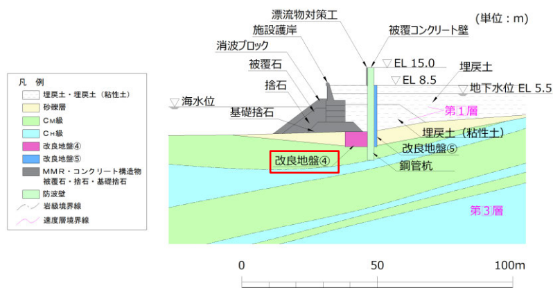
図 4.2-2 改良地盤④の配置図
