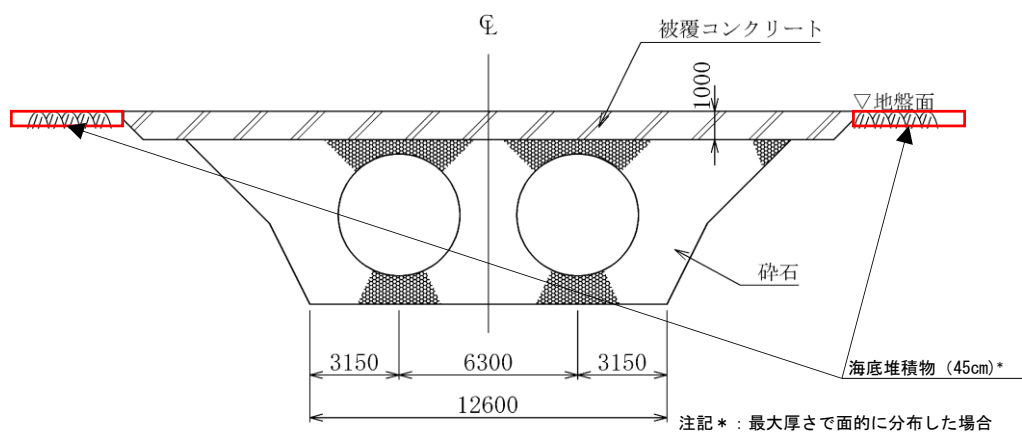
図 4-6 取水口断面図
