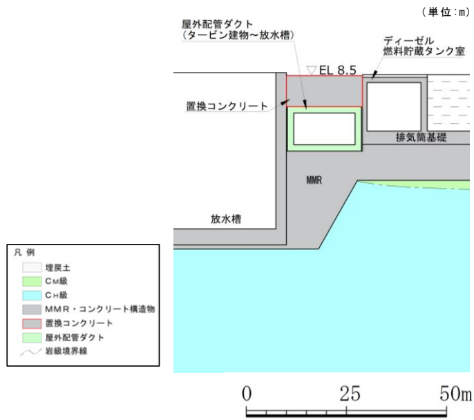
図 4.7-2 置換コンクリートの配置図
