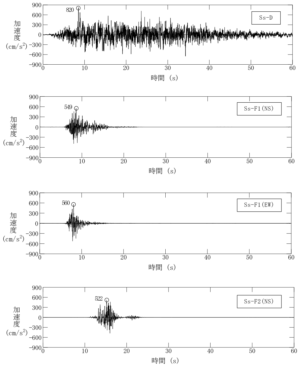
図 2-3 基準地震動の加速度時刻歴波形（水平方向） (S s - D, S s - F 1 (N S), S s - F 1 (E W), S s - F 2 (N S))
