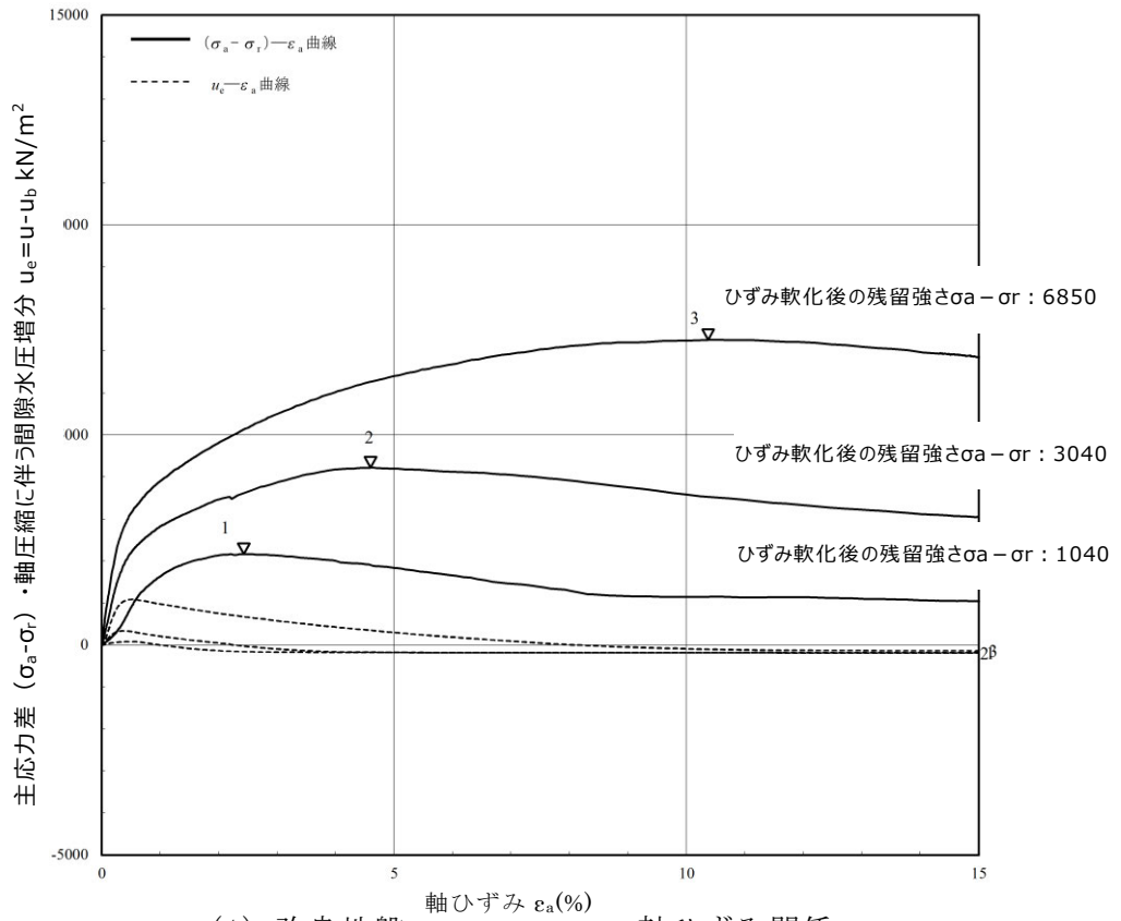
(1) 改良地盤 - 軸ひずみ関係
