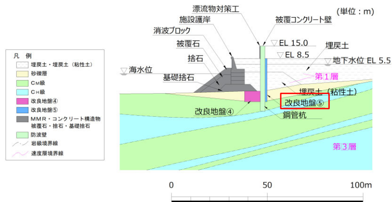
図 4.3-2 改良地盤⑤の配置図
