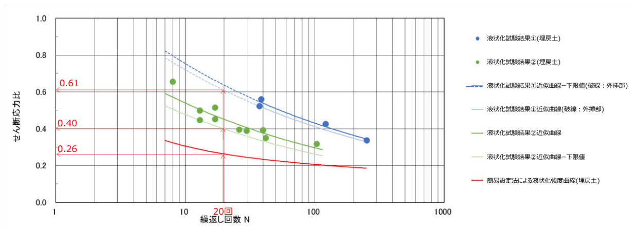
図 2-1 簡易設定法及び液状化強度試験結果による液状化強度曲線の比較（埋戻土）
