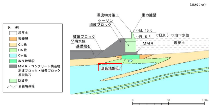
図 4.4-2 改良地盤⑥の配置図
