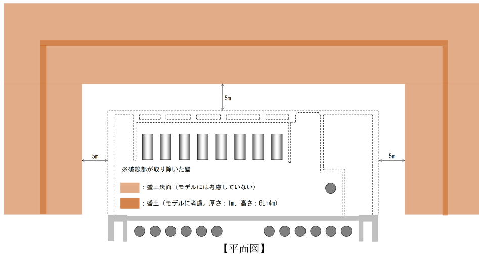
第 5-3 図 貯蔵建屋壁の遮蔽機能喪失の仮定
