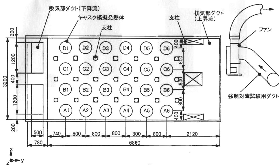
別添 1 - 6 図 試験装置の貯蔵部平面図 1)
