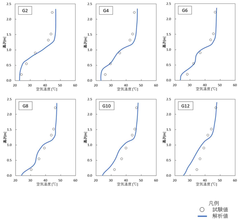
別添 1 - 13 図 建屋内温度分布 (その 3)
