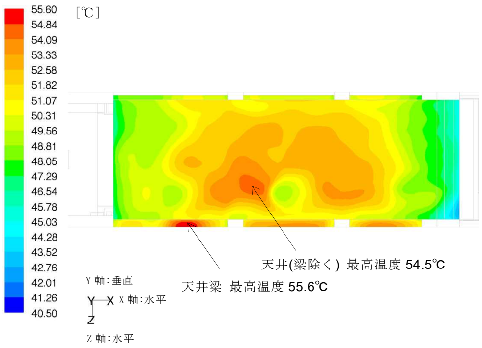
第 10-3 図 天井表面温度分布
