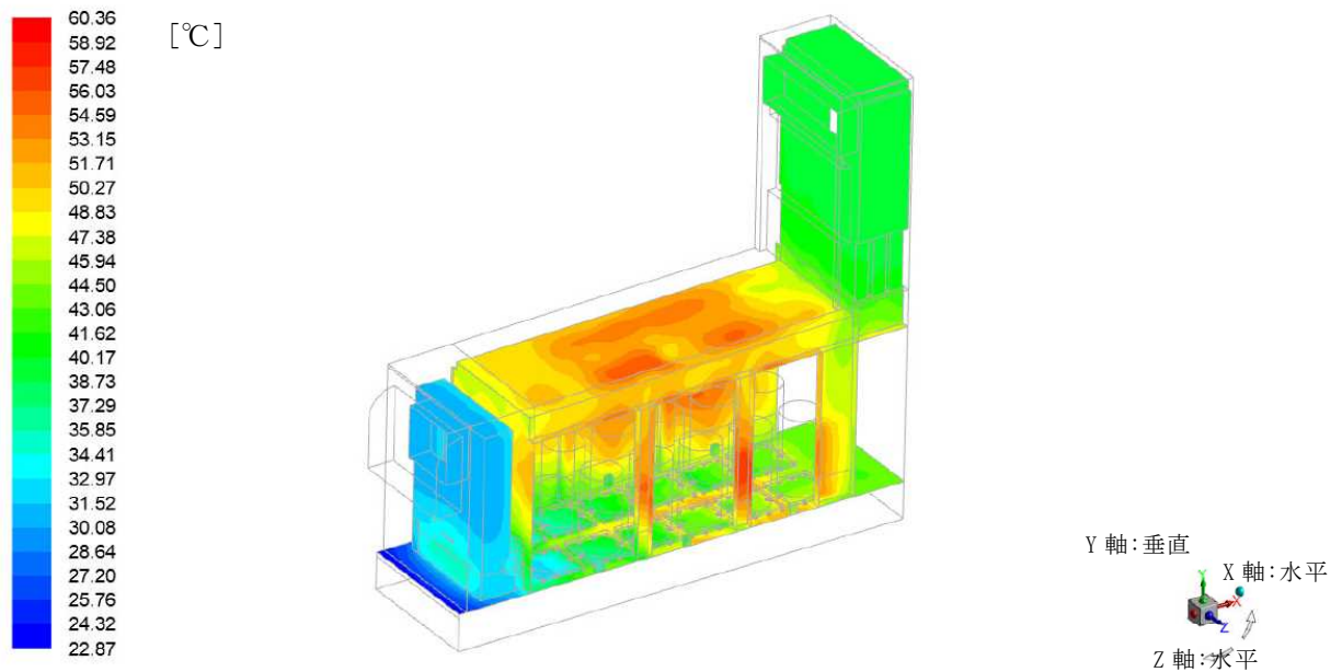
第 12-1 図 躯体全体 (床・側壁・天井・支柱) 表面温度分布 (PWR用キャスク(タイプ1))
