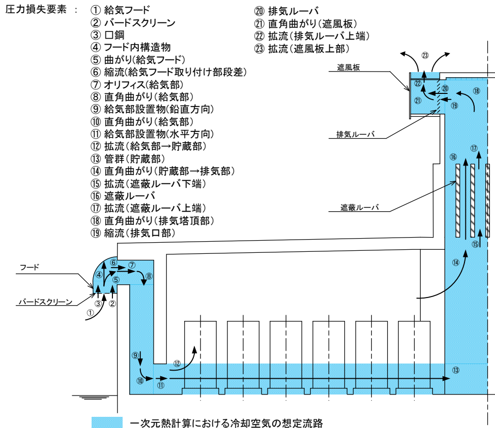
第5図 一次元熱計算における流路設定及び考慮する圧力損失要素
