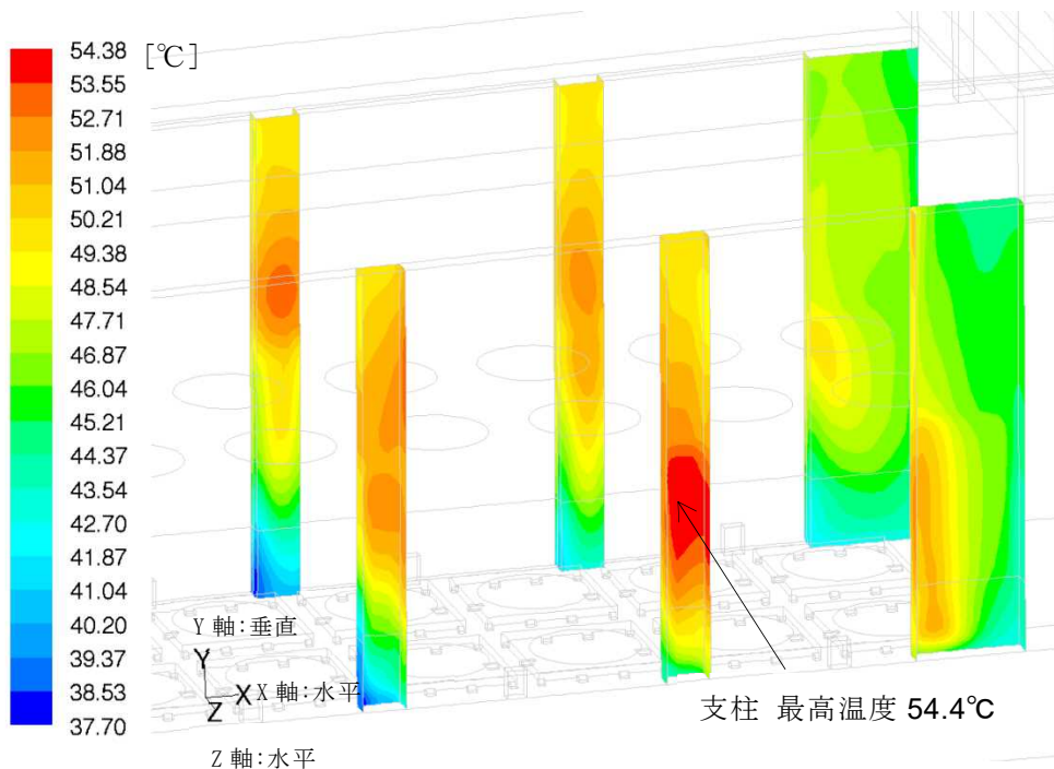
第 10-4 図 支柱表面温度分布
