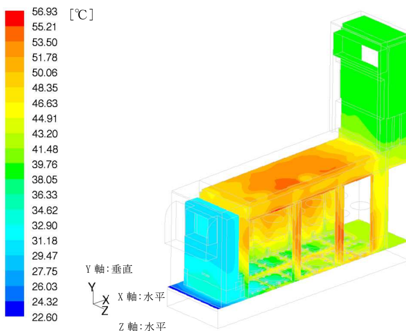
第10-1図 躯体全体(床・側壁・天井・支柱)表面温度分布
