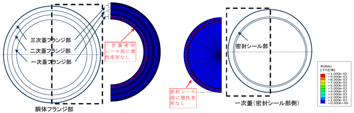
第 4-3-3 図 (3/3) 天井クレーン落下時の水平姿勢キャスクのひずみ評価結果 (PWR用キャスク (タイプ1) の場合)
