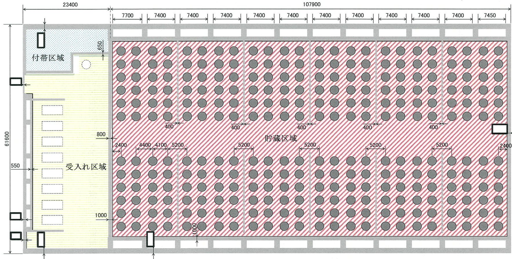
別添4-1図 貯蔵建屋内の遮蔽設計区分
