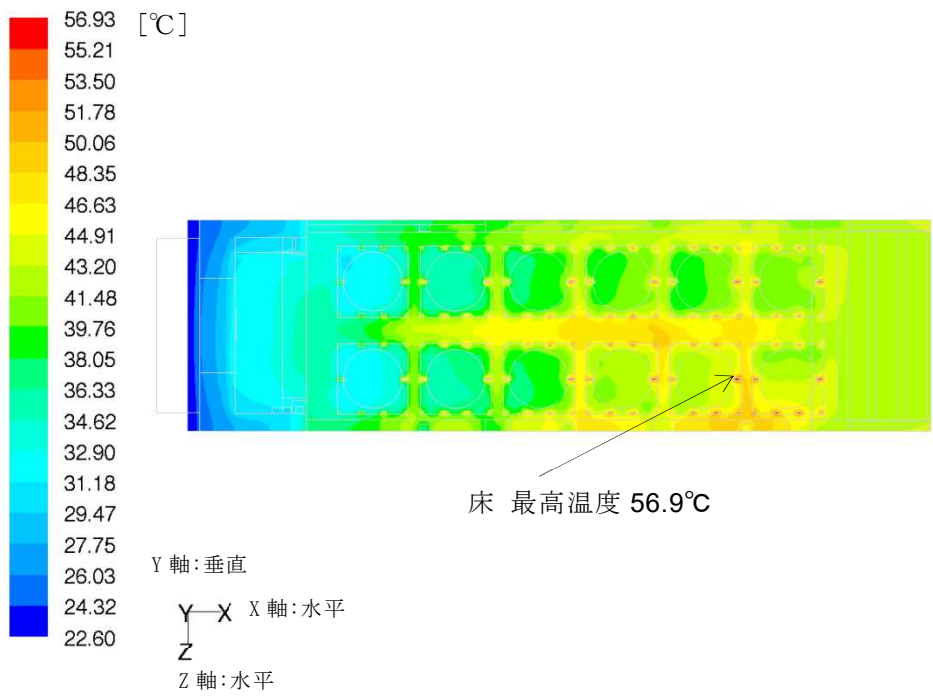
第 10-2 図 床表面温度分布
