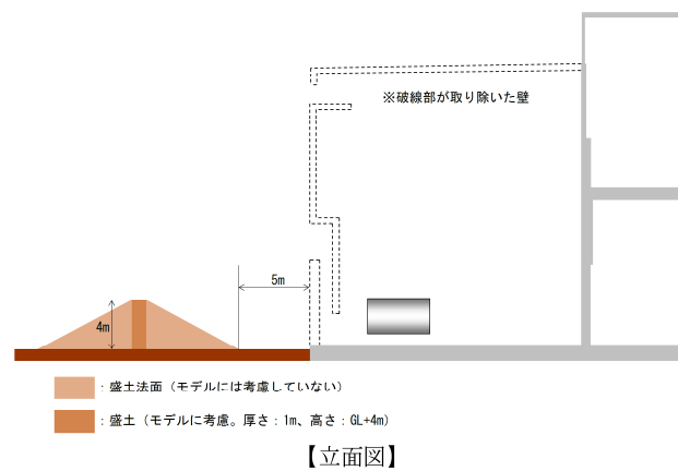
第 5-4 図 盛土のイメージ図
