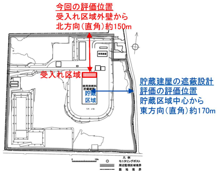
第 5-5 図 線量評価位置
