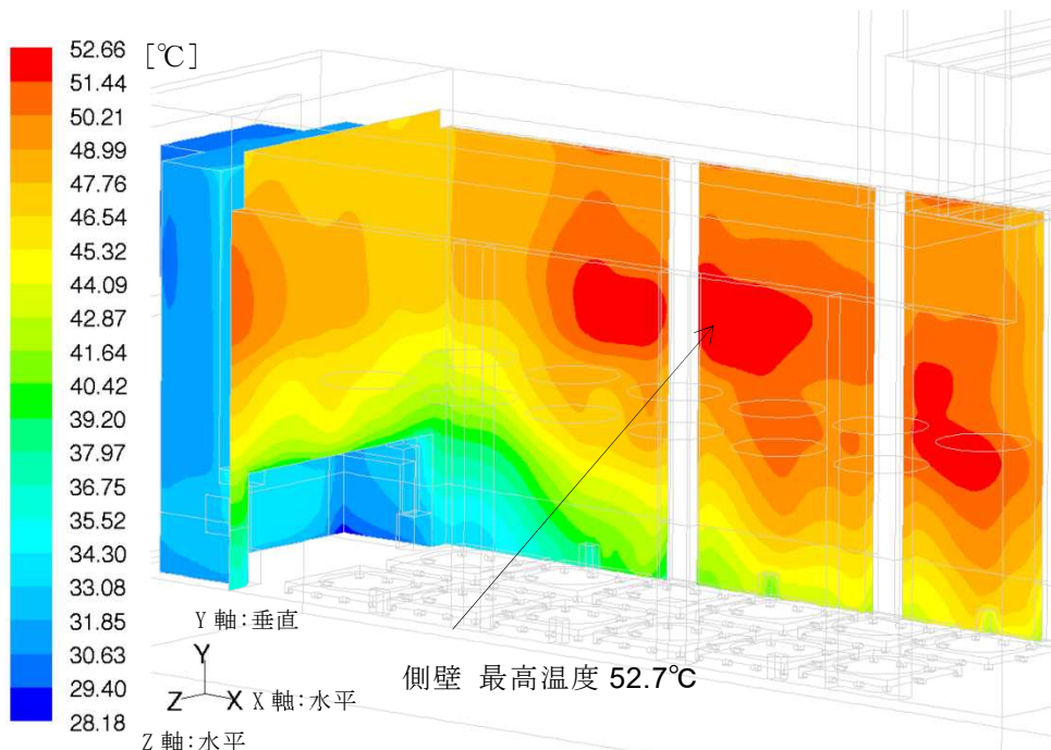
第 10-5 図 側壁・入口壁表面温度分布
