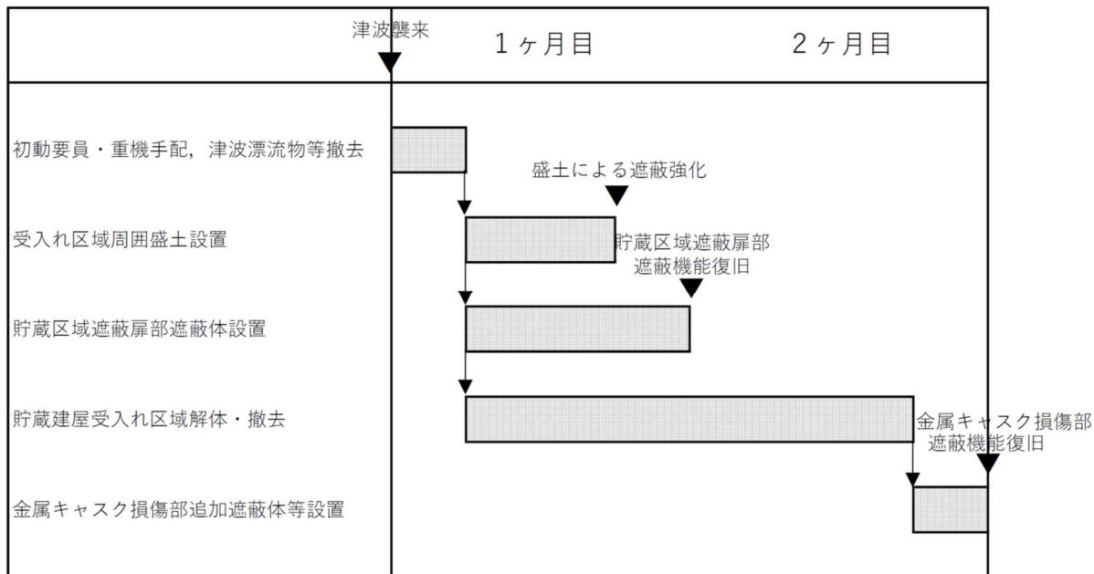
別添7図 遮蔽機能復旧工程（想定）
