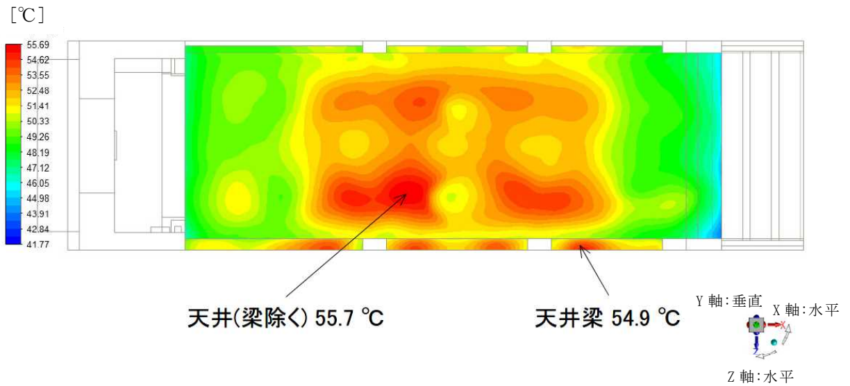
第 11-5 図 天井表面温度分布 (BWR用中型キャスク(タイプ2))
