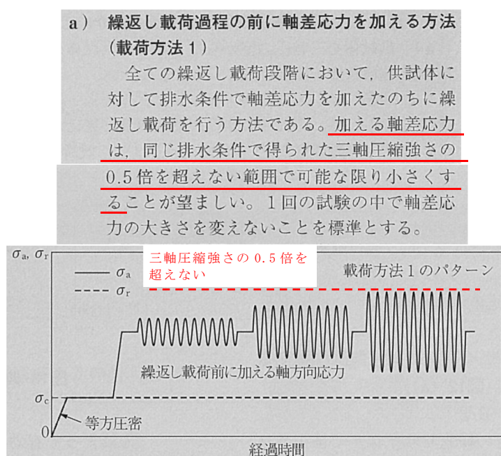
図 4.5.3-4 JGS 2563 载荷方法の模式図等(赤字で加筆) (参考) 13-78
