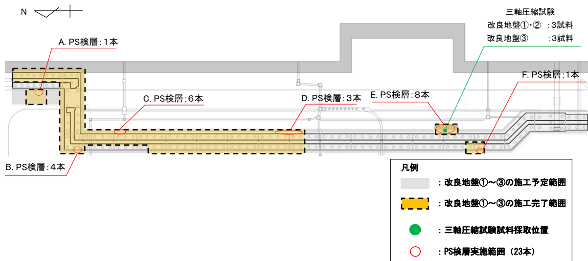
図 5.5.1-1 改良地盤①～③の品質確認のために実施する原位置試験及び試料採取位置
