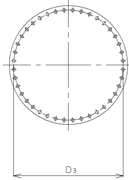
C~C 矢視図
