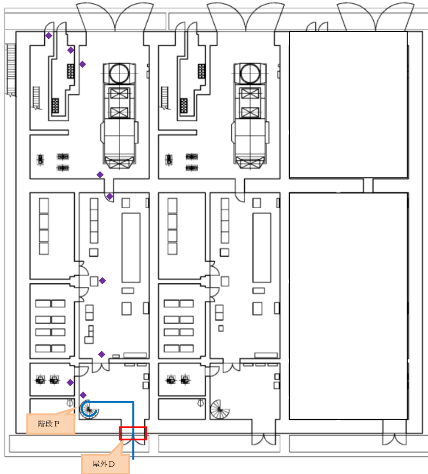
図 4-2 屋内アクセスルート図(9/11)
