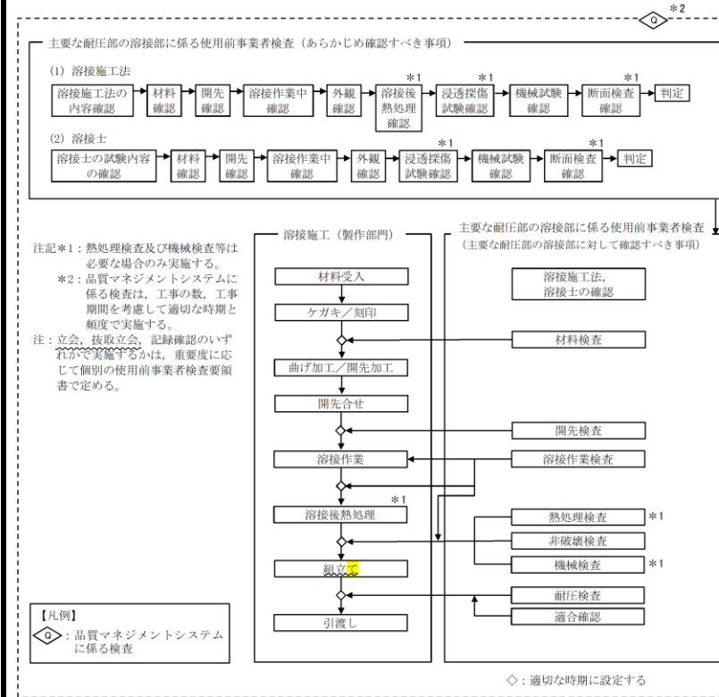
図1-2 主要な耐圧部の溶接部に係る工事の手順と使用前事業者検査フロー
