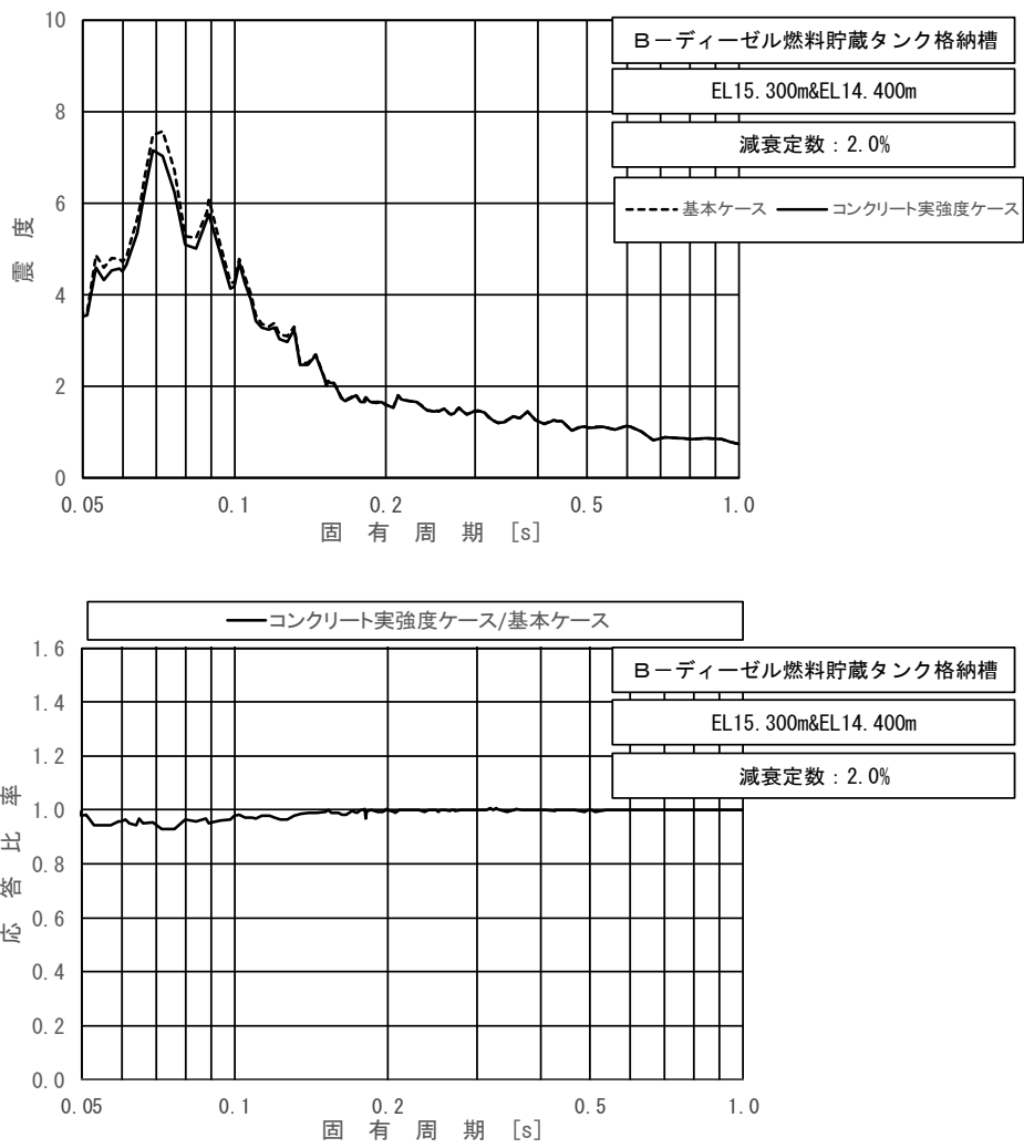
図 3.1.3-3(2/4) 床応答スペクトル (B-ディーゼル燃料貯蔵タンク格納槽) (基準地震動 S_s - D (++) , 鉛直方向, EL15.300~14.400m, 減衰 2.0%)
