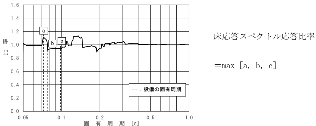
図 2.2-1 簡易評価に用いる各方向における床応答スペクトルの応答比率の適用方法 （評価に床応答スペクトルを適用する設備）
