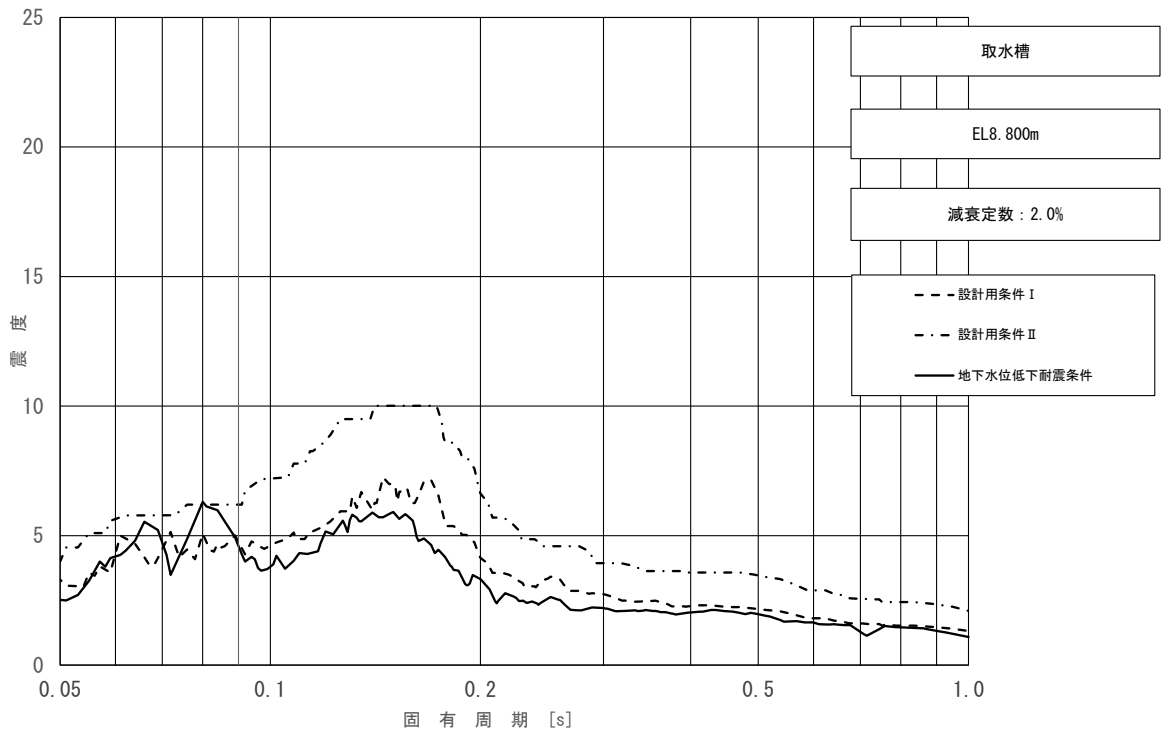
図 3.2.1-2(1/3) 地下水位低下床応答スペクトル (取水槽 (海水ポンプエリア)) (水平方向 (E W 方向), EL8.800m, 減衰 2.0%)
