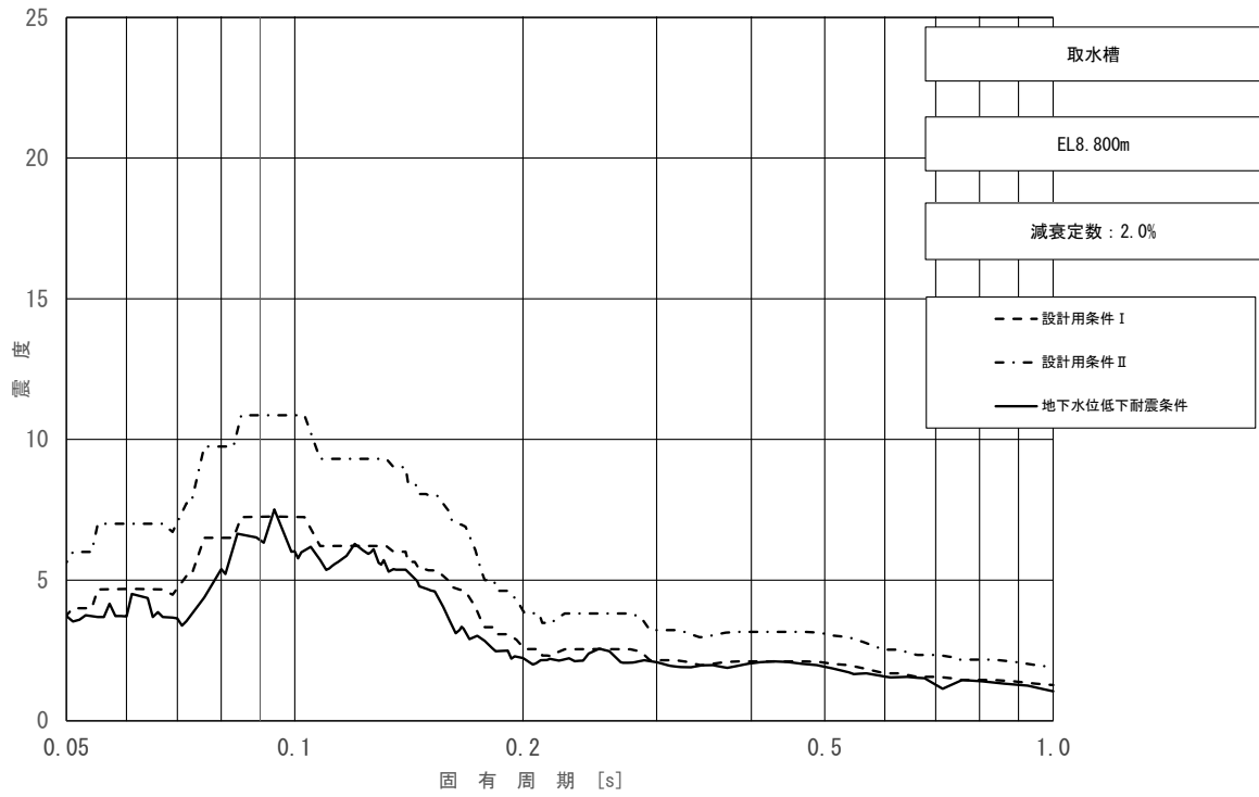
図 3.2.1-1(1/3) 地下水位低下床応答スペクトル (取水槽 (海水ポンプエリア)) (水平方向 (N S 方向), EL. 800m, 減衰 2.0%)
