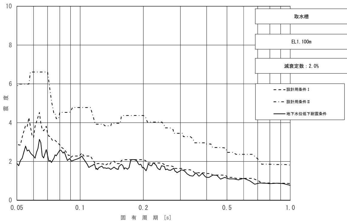
図 3.2.1-3(2/3) 地下水位低下床応答スペクトル (取水槽 (海水ポンプエリア)) (鉛直方向, EL. 100m, 減衰 2.0%)
