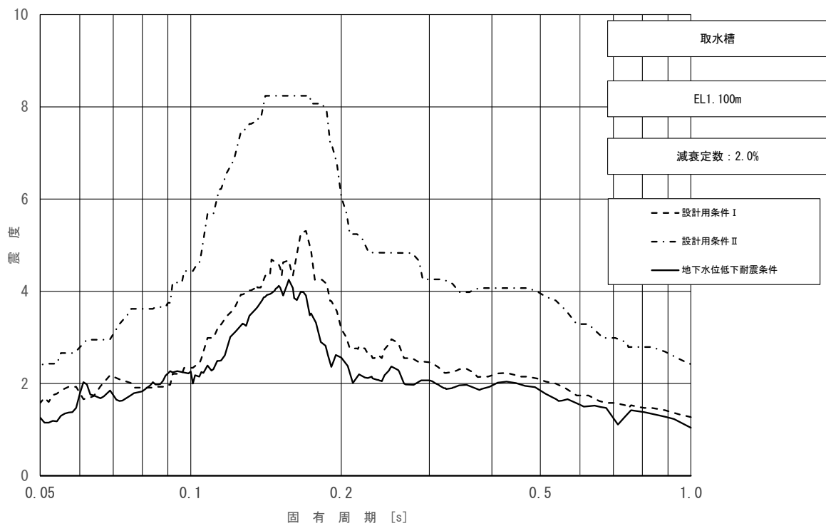
図 3.2.1-2(2/3) 地下水位低下床応答スペクトル (取水槽 (海水ポンプエリア)) (水平方向 (EW方向), EL1.100m, 減衰 2.0%)
