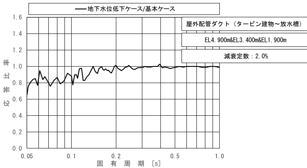
図 3.1.5-6 床応答スペクトル (屋外配管ダクト (タービン建物～放水槽) (EW断面)) (基準地震動 S s - D (++) , 鉛直方向, EL4.900m~EL1.900m, 減衰 2.0%)
