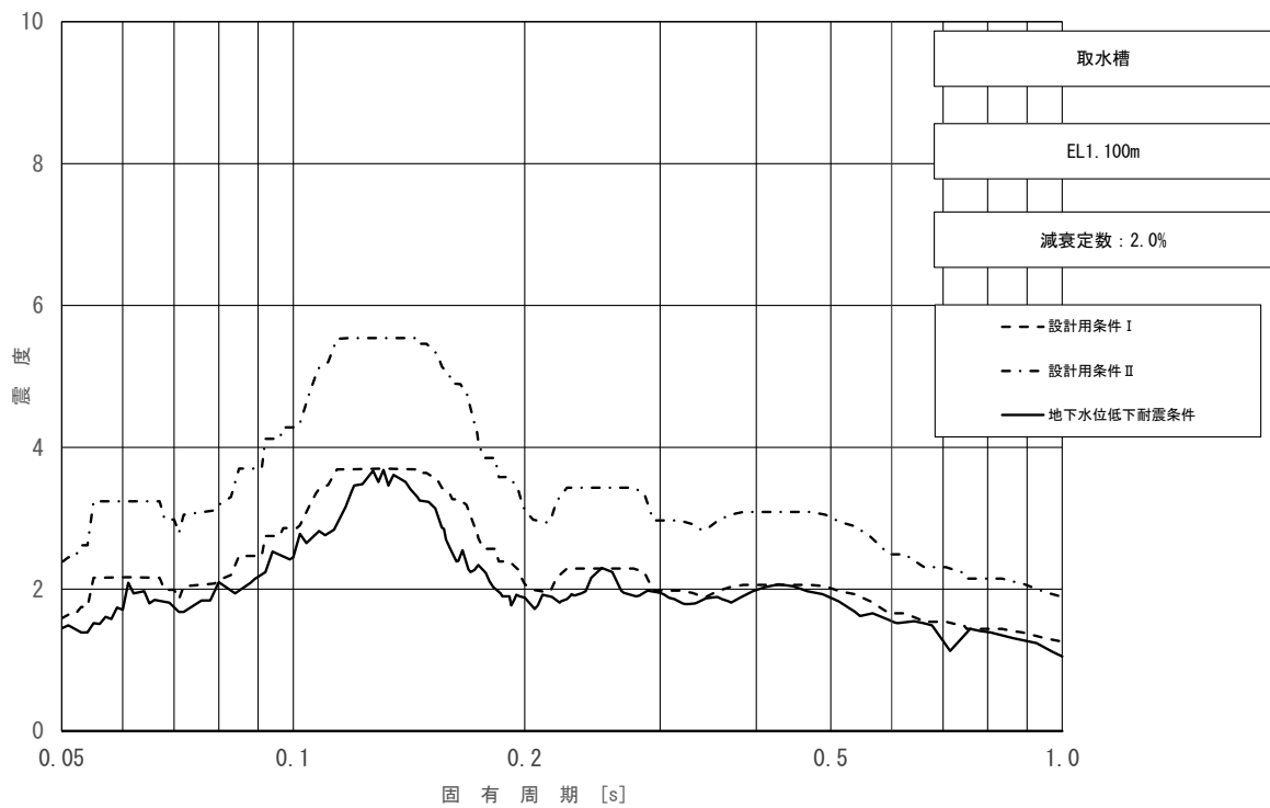
図 3.2.1-1(2/3) 地下水位低下床応答スペクトル (取水槽 (海水ポンプエリア)) (水平方向 (N S 方向), EL. 100m, 減衰 2.0%)
