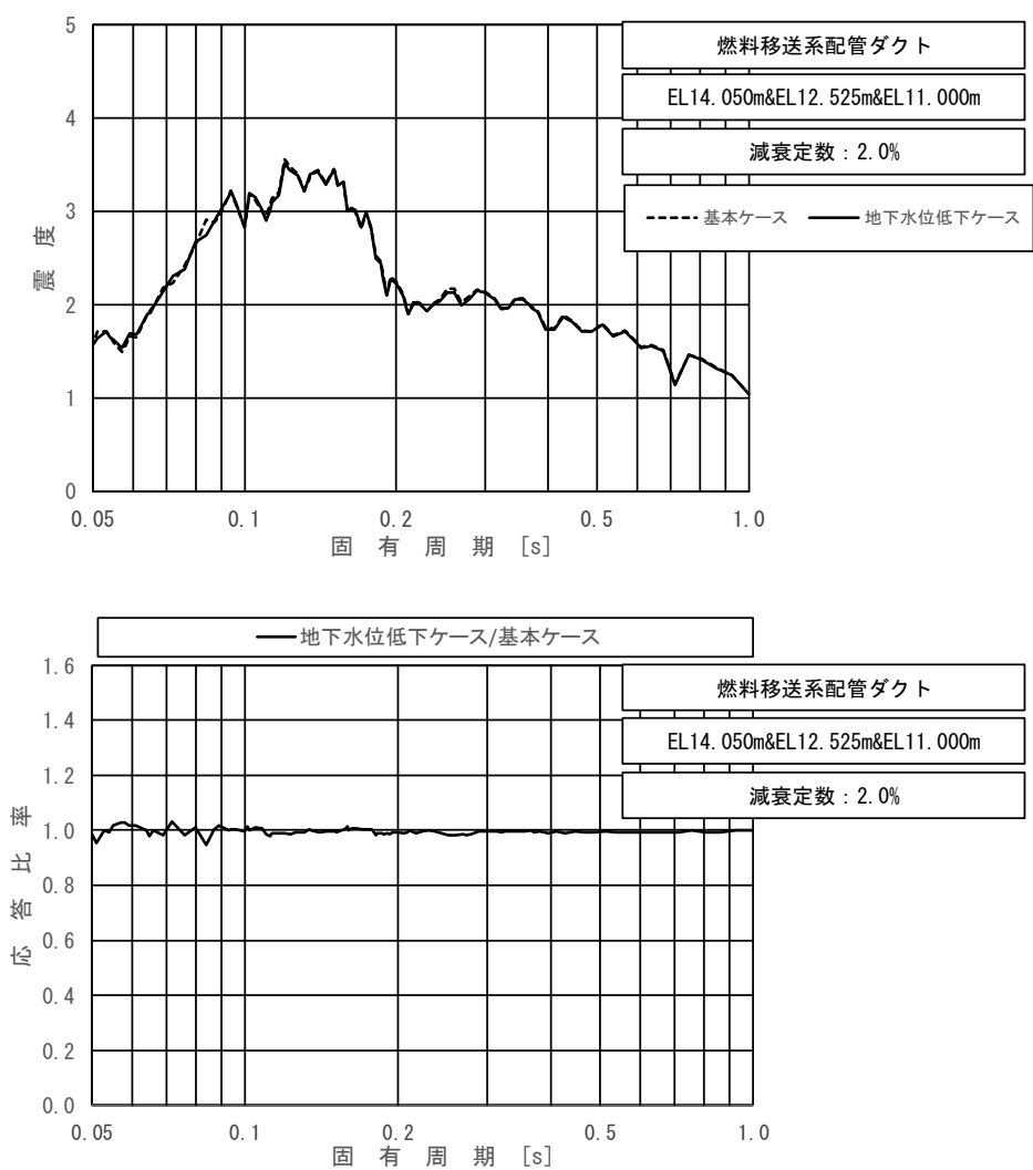
図 3.1.4-5 床応答スペクトル (屋外配管ダクト (B-ディーゼル燃料貯蔵タンク～原子炉建物) (燃料移送系配管ダクト))
