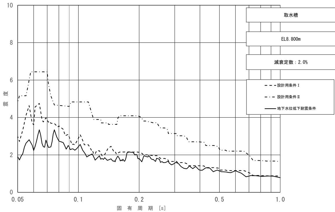
図 3.2.1-3(1/3) 地下水位低下床応答スペクトル (取水槽 (海水ポンプエリア)) (鉛直方向, EL. 800m, 減衰 2.0%)
