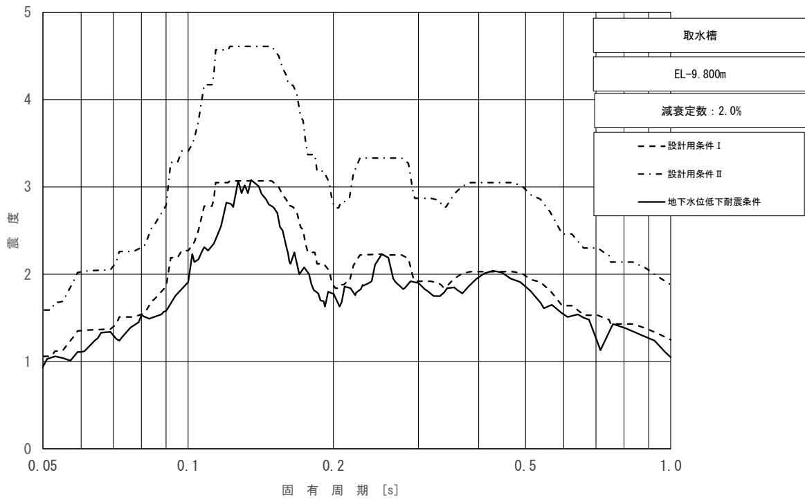
図 3.2.1-1(3/3) 地下水位低下床応答スペクトル (取水槽 (海水ポンプエリア)) (水平方向 (N S 方向), EL-9.800m, 減衰 2.0%)
