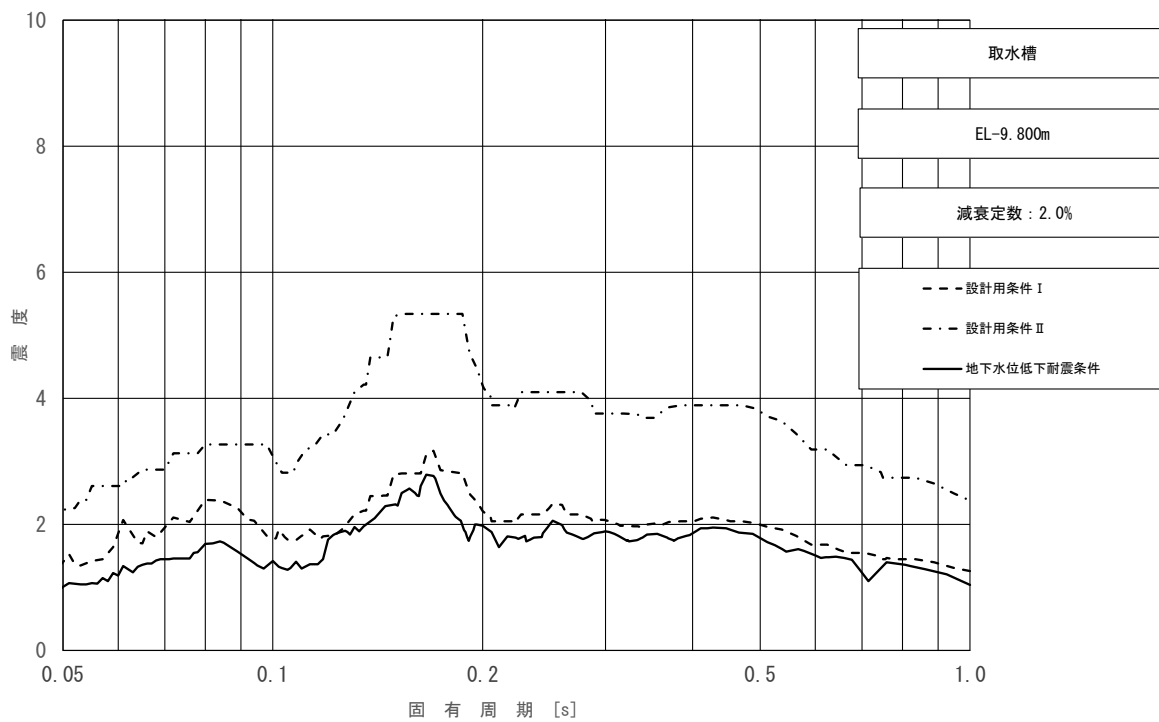
図 3.2.1-2(3/3) 地下水位低下床応答スペクトル (取水槽 (海水ポンプエリア)) (水平方向 (EW方向), EL-9.800m, 減衰 2.0%)
