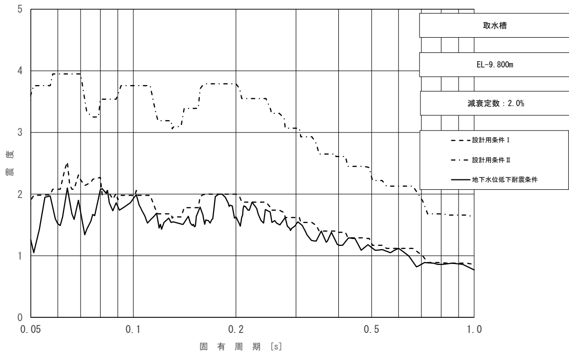
図 3.2.1-3 (3/3) 地下水位低下床応答スペクトル (取水槽 (海水ポンプエリア)) (鉛直方向, EL-9.800m, 減衰 2.0%)
