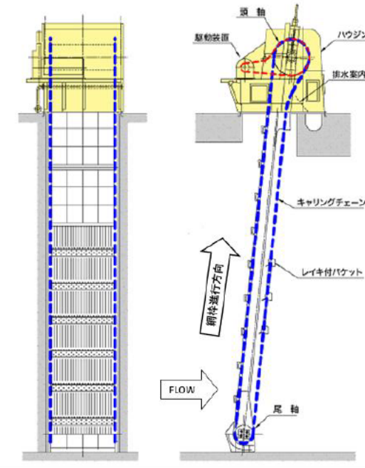
図 3-39 除じん機の概要
