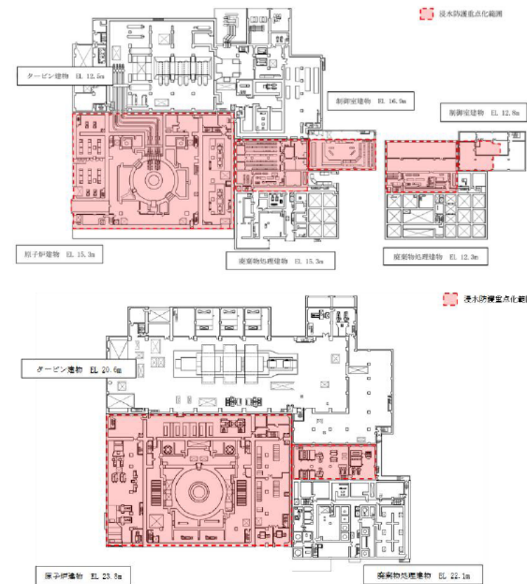
図 3-29(2) 浸水防護重点化範囲 (平面図) (2/4)
