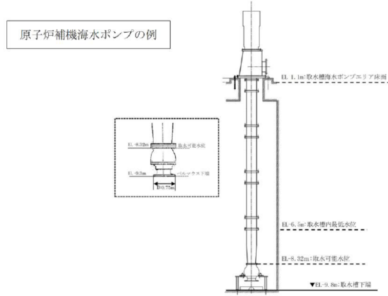
図 3-37 原子炉補機海水ポンプの取水可能水位
