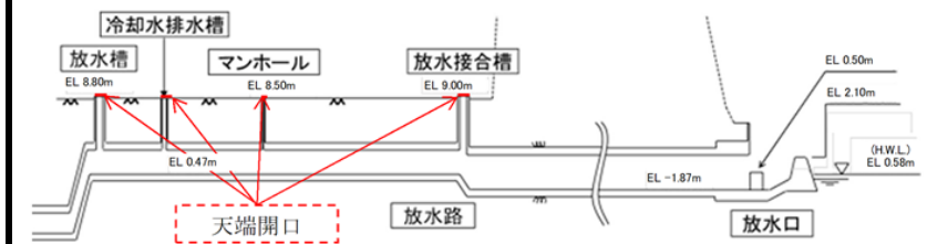
図 3-20 1号機 放水施設の断面図
