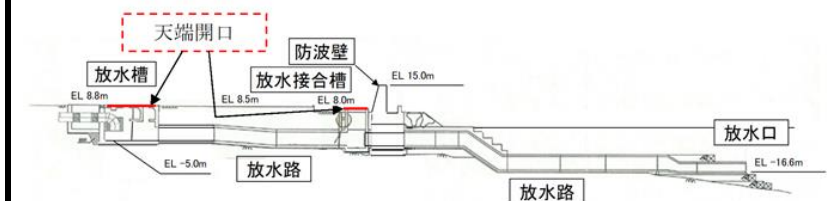
図 3-21 3号機 放水施設の断面図
