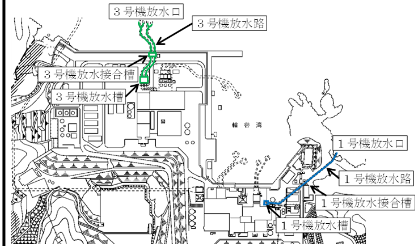
図 3-19 1, 3号機 放水施設の配置図
