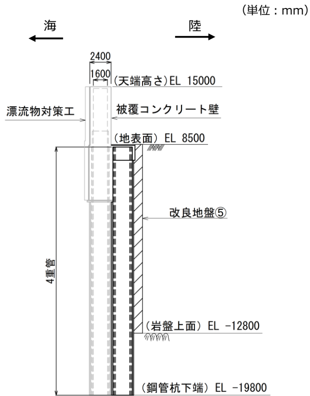
(断面図)
