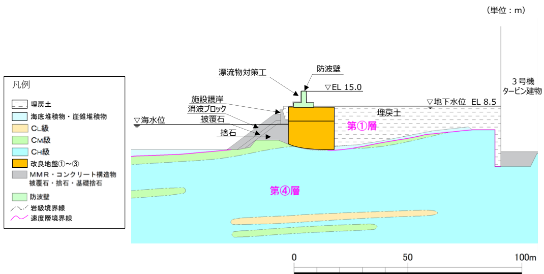
図 1.8.2-48 影響確認断面の地質断面図（⑤-⑤断面）
