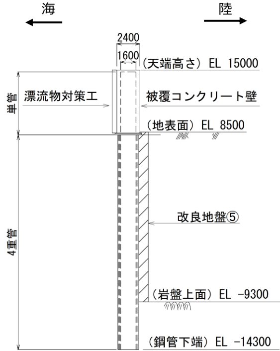
(断面図)
