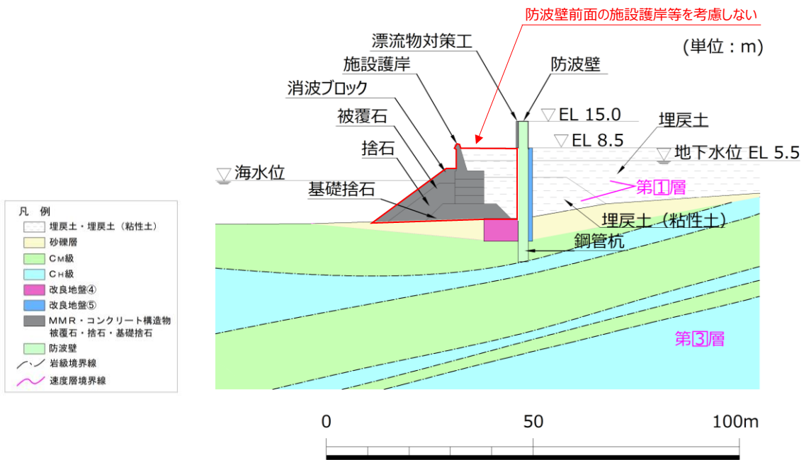
図 1.8.2-23 施設護岸等が損傷した場合の影響確認断面（②-②断面）
