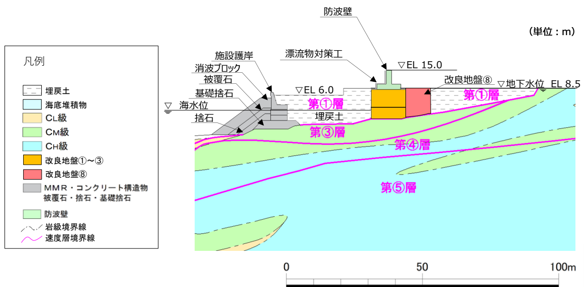
図 1.8.2-46 改良地盤⑧影響検討断面図（①-①断面）
