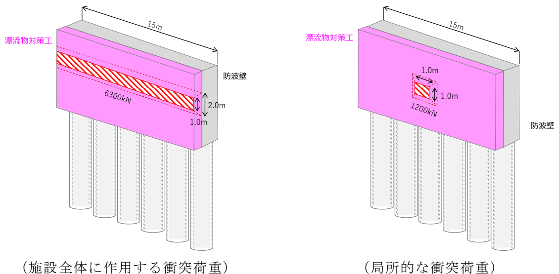
図 1.5.1-12 防波壁（多重鋼管杭式擁壁）の漂流物衝突荷重の载荷イメージ
