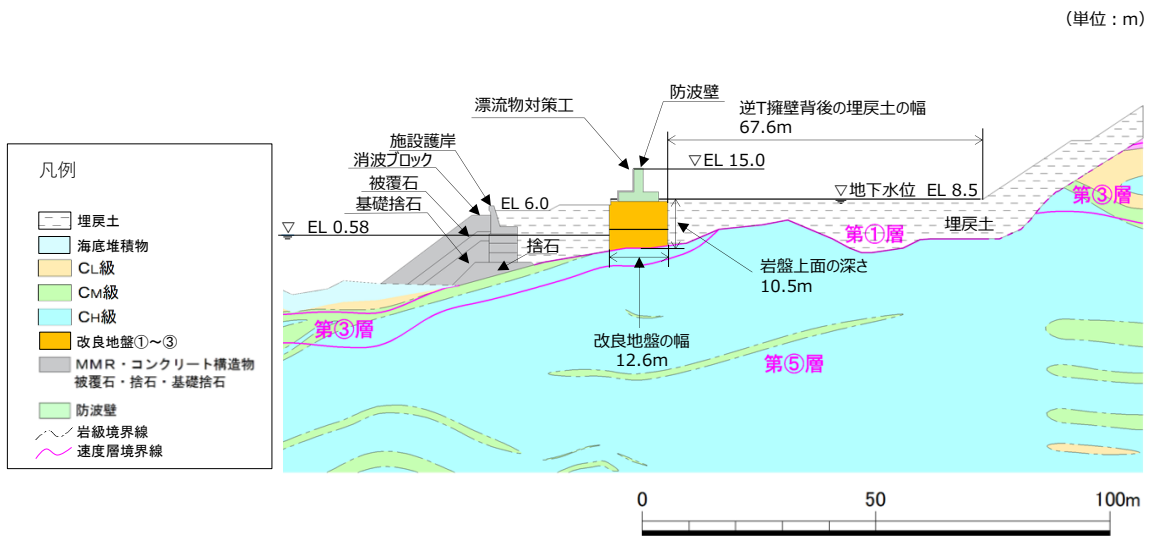
図 1.8.2-32 防波壁（逆T擁壁）の横断面図（②-②断面）
