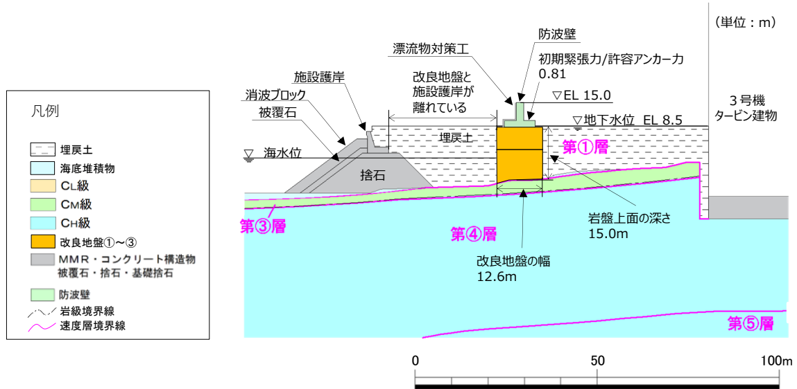
図 1.8.2-34 防波壁（逆T擁壁）の横断面図（④-④断面）
