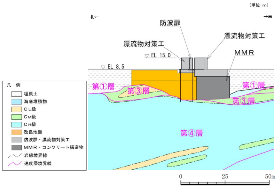
図 1.8.3-6(2) 防波壁通路防波扉（3号機東側） A-A断面図
