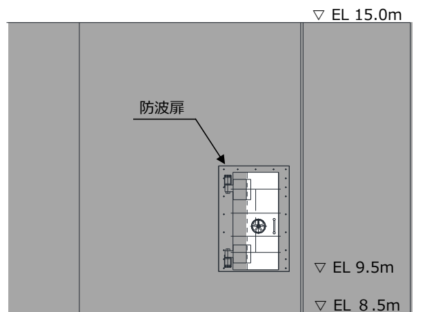
图 1.8.3-4(3) 防波壁通路防波扉（2号機北側） B-B 断面图
