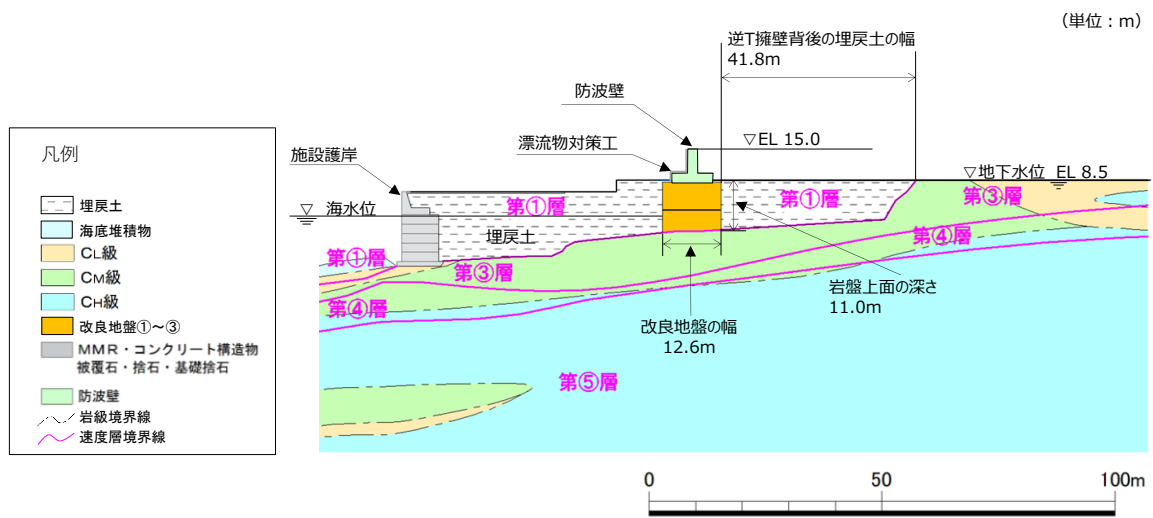
図 1.8.2-36 防波壁（逆T擁壁）の横断面図（⑥-⑥断面）
