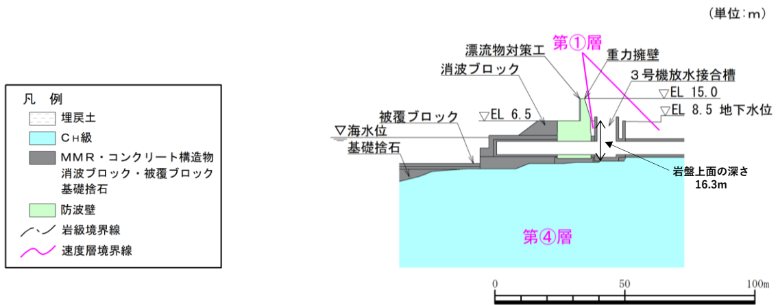
図 1.8.2-57 防波壁（波返重力擁壁）の横断面図 放水路貫通部（③-③断面）
