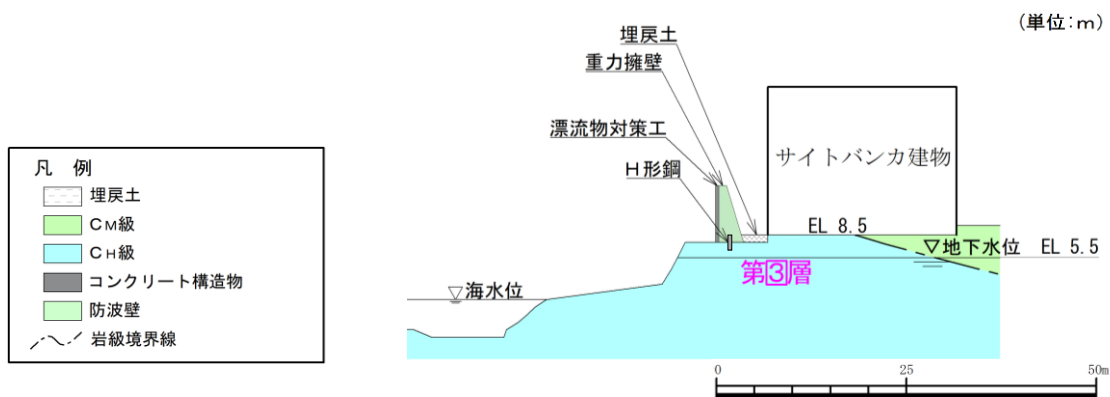
図 1.8.2-59 防波壁（波返重力擁壁）の横断面図 東端部（⑤-⑤断面）
