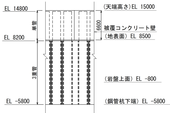
(正面図)
