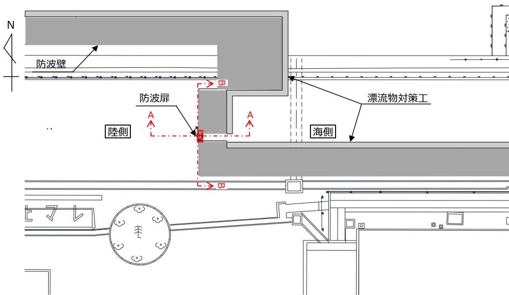
图 1.8.3-4(1) 防波壁通路防波扉（2号機北側） 平面图
