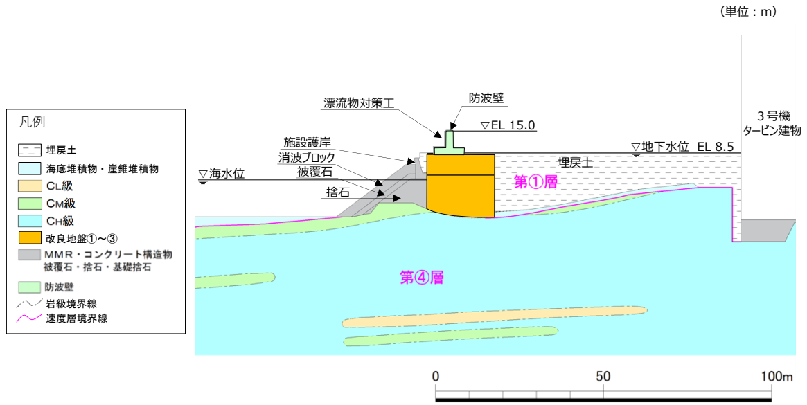
図 1.8.2-35 防波壁（逆T擁壁）の横断面図（⑤-⑤断面）
