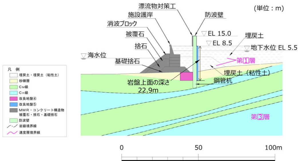
図 1.8.2-9 防波壁（多重鋼管杭式擁壁）の横断面図 改良地盤部（②-②断面）
