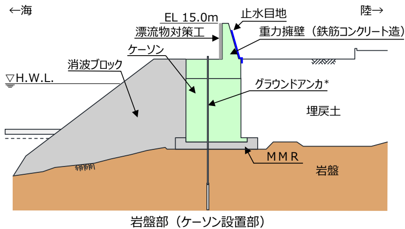
図 1.6.2-48 防波壁の断面図
