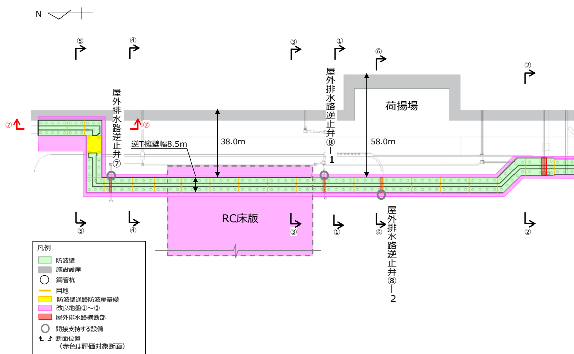
図 1.8.2-41 評価対象断面（縦断方向）の平面位置図
