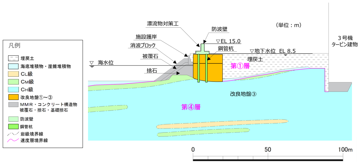
図 1.8.2-44 鋼管杭影響検討断面図 (⑤-⑤断面)
