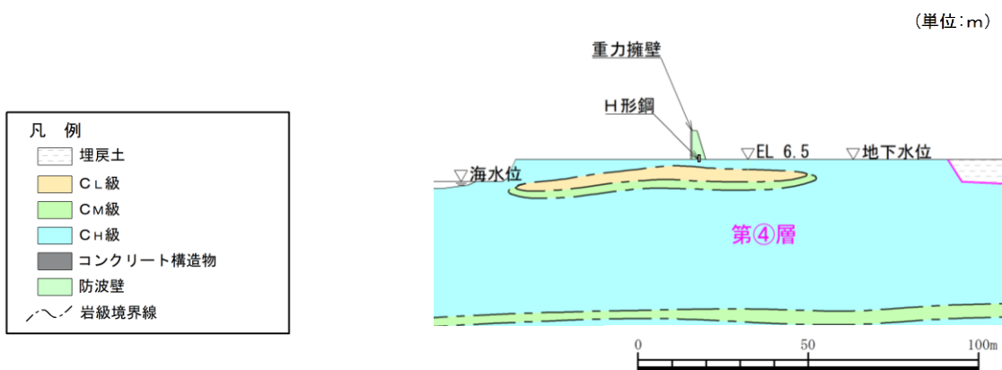
図 1.8.2-60 防波壁（波返重力擁壁）の横断面図 西端部（⑥-⑥断面）
