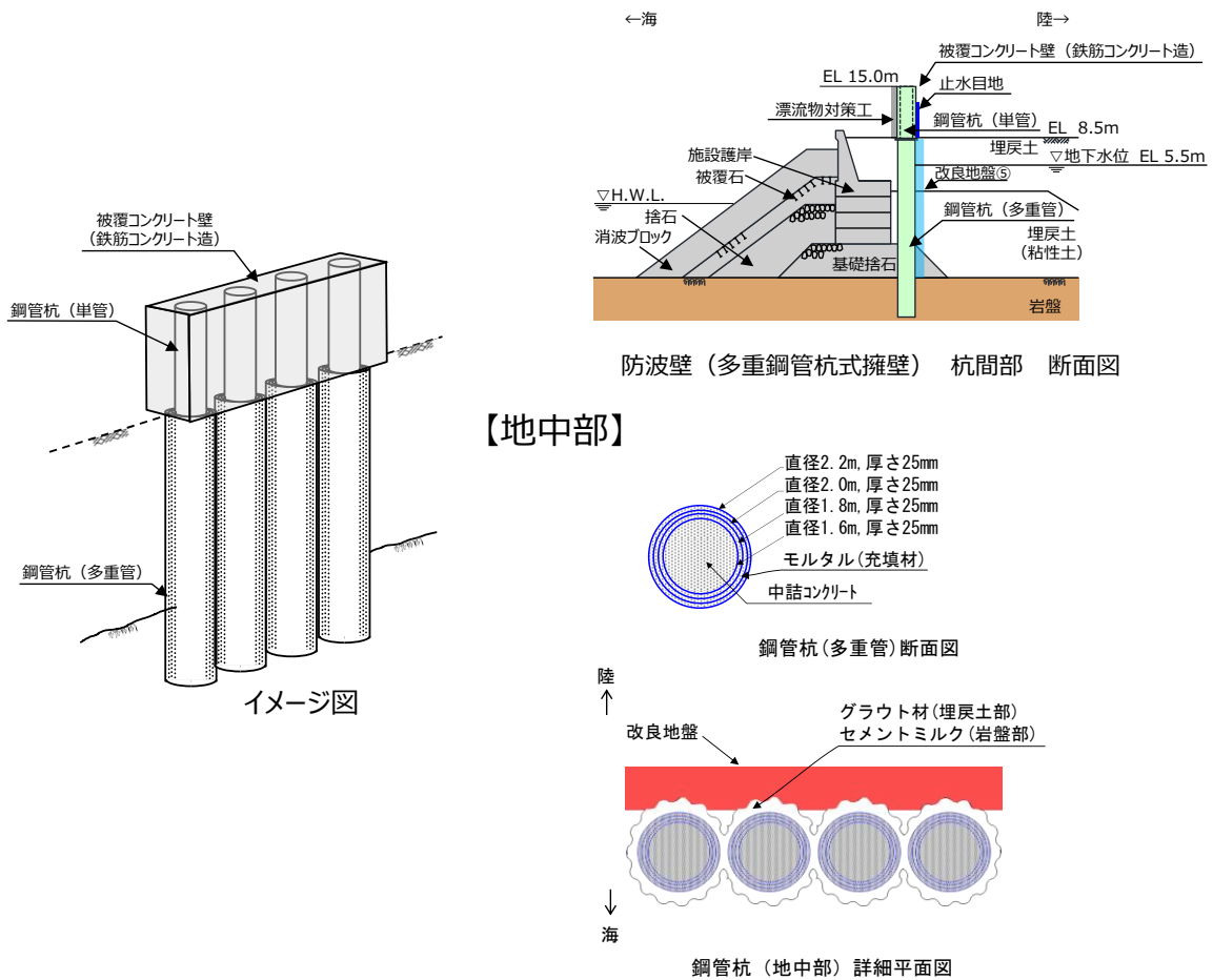
図 1.8.2-5 防波壁 (多重鋼管杭式擁壁) の構造概要図 (断面図)
