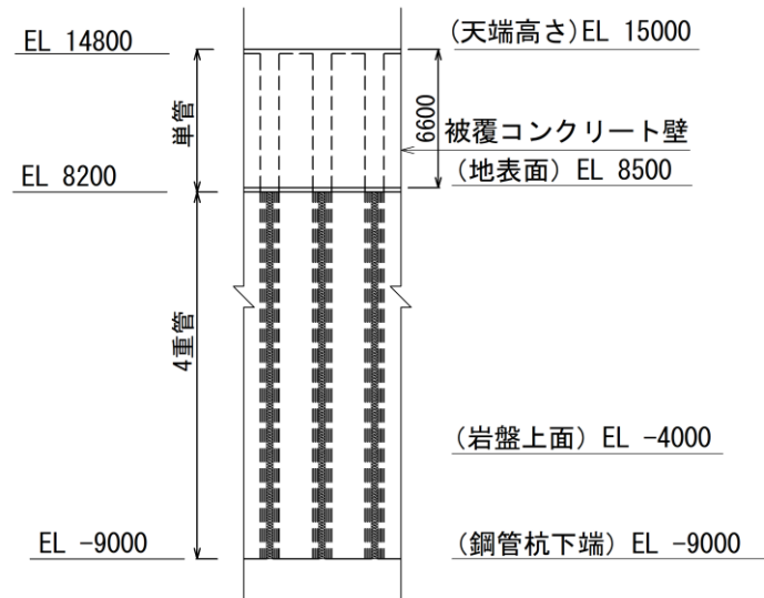
(正面図)
