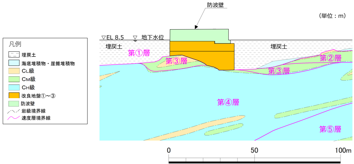
図 1.8.2-37 防波壁（逆T擁壁）の横断面図（⑦-⑦断面）
