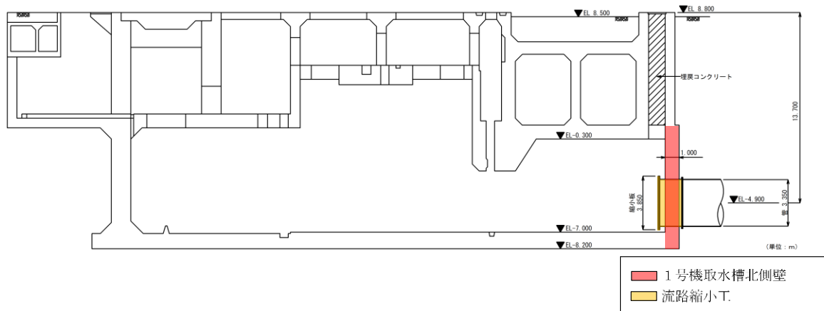
(1号機取水槽 縦断図)
