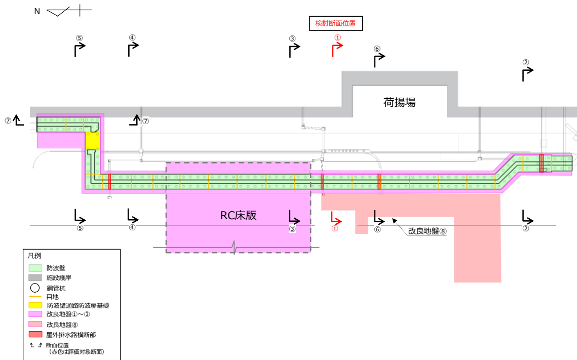
図 1.8.2-45 改良地盤⑧の位置図
