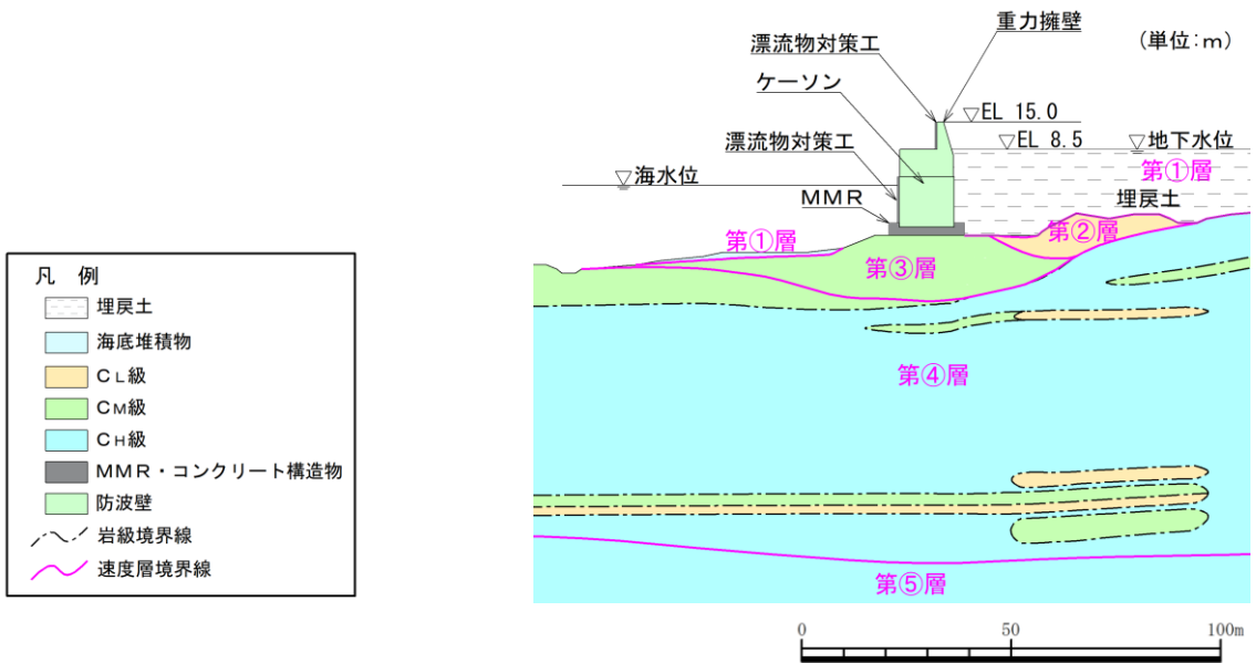
図 1.8.2-58 防波壁（波返重力擁壁）の横断面図 輪谷部（④-④断面）
