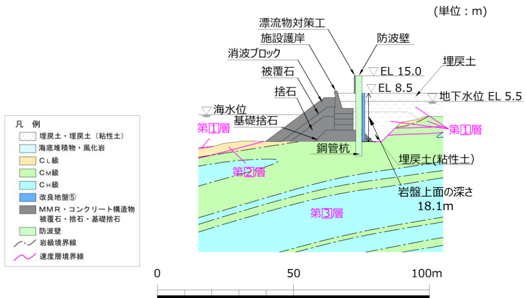
図 1.8.2-8 防波壁（多重鋼管杭式擁壁）の横断面図 一般部（①-①断面）
