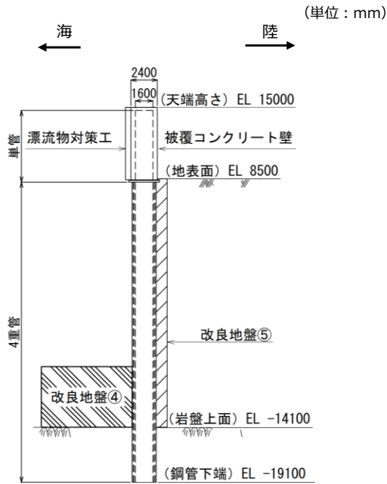
(断面図)
