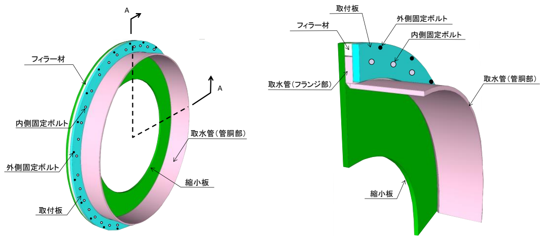
(流路縮小工 鳥瞰図)
