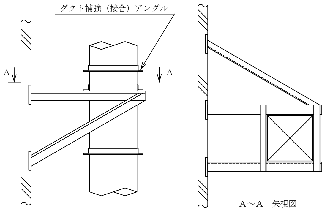
図3-7 垂直ダクトの支持の代表例（2方向（軸直角方向）拘束の代表例）
