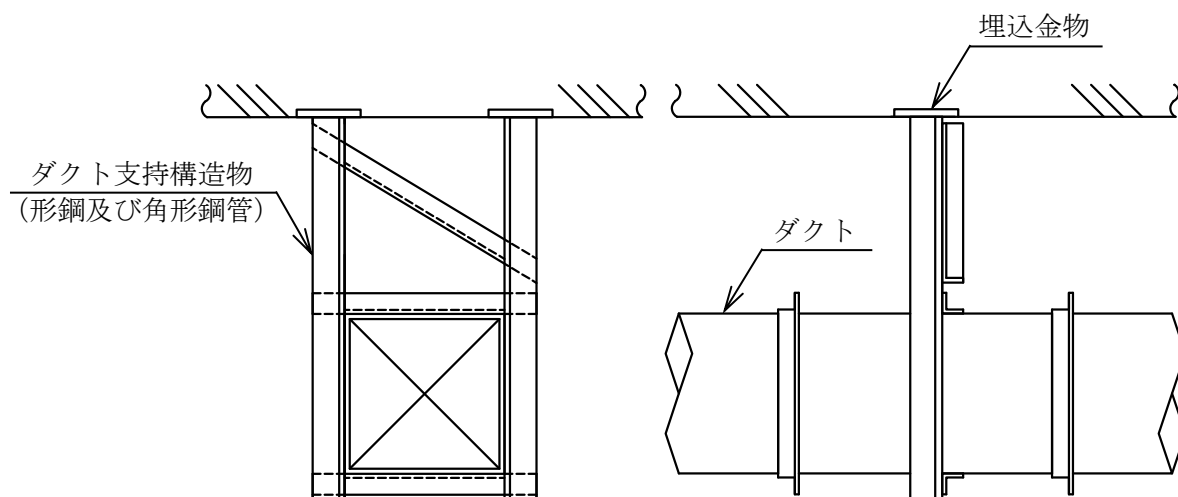
図 3-5 2方向（軸直角方向）拘束の代表例
