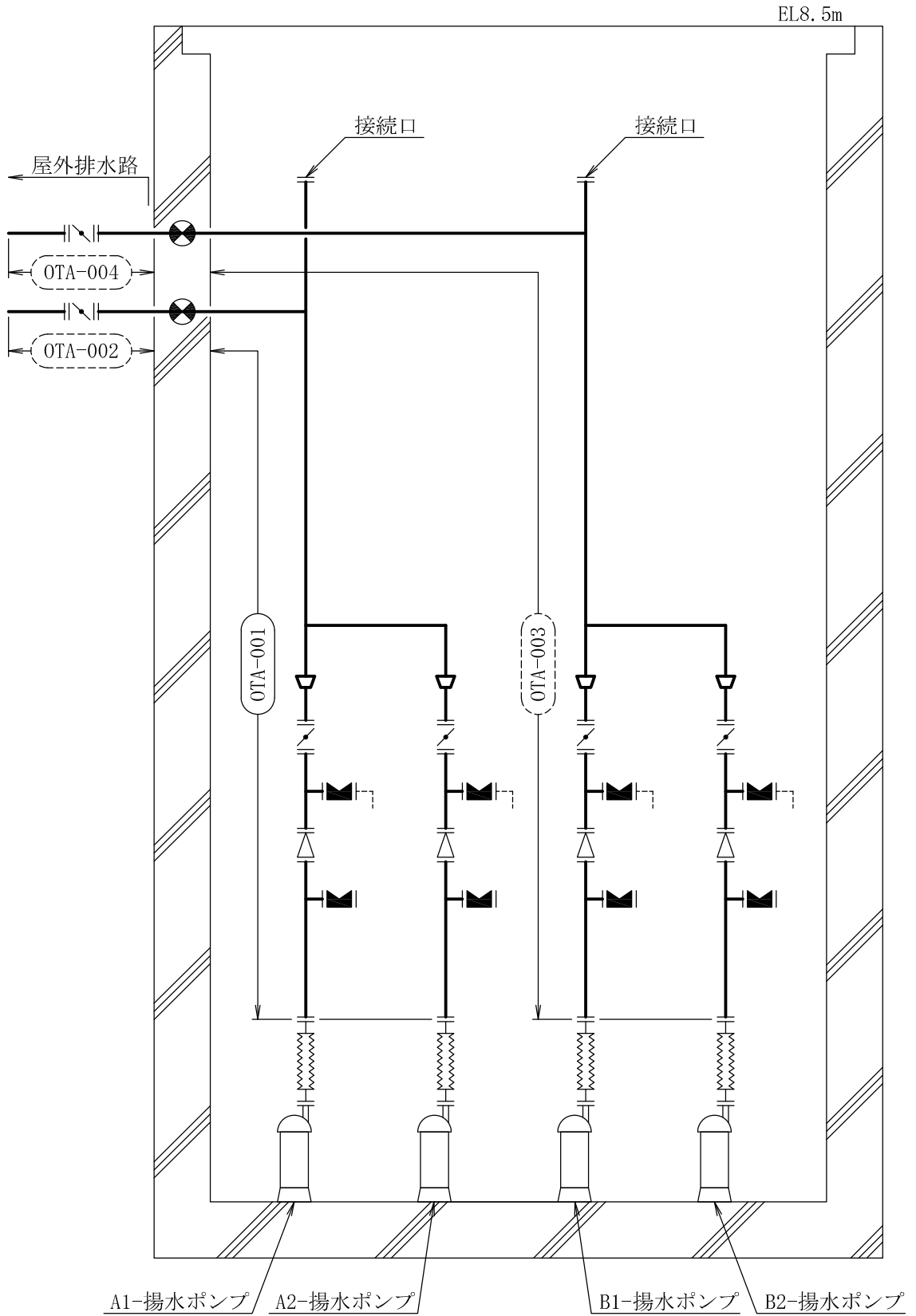
地下水水位低下設備概略系統図
