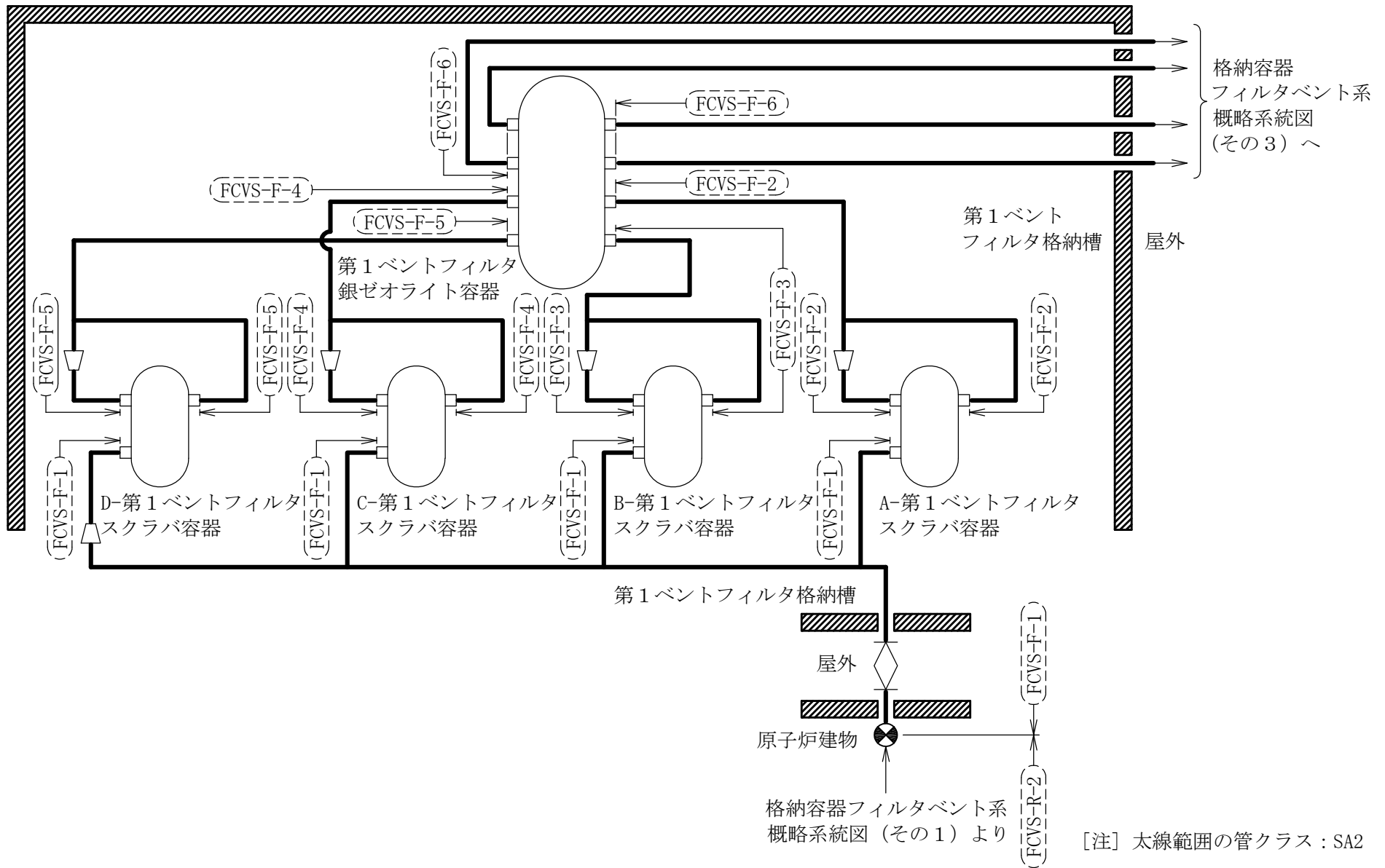
格納容器フィルタベント系概略系統図 (その2)
