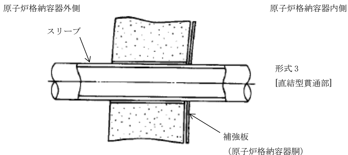
図 2-1 配管貫通部の形式
