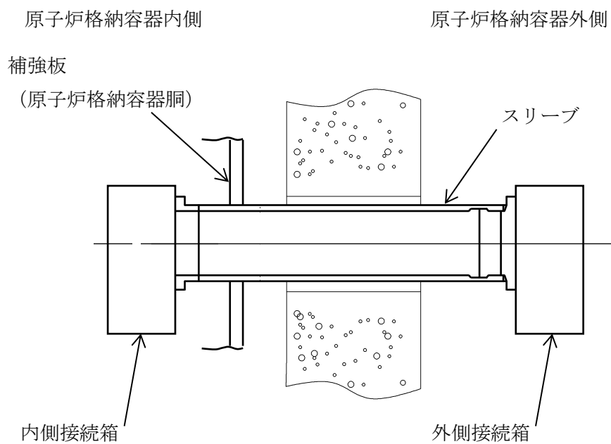
図 2-2 電気配線貫通部の形式
