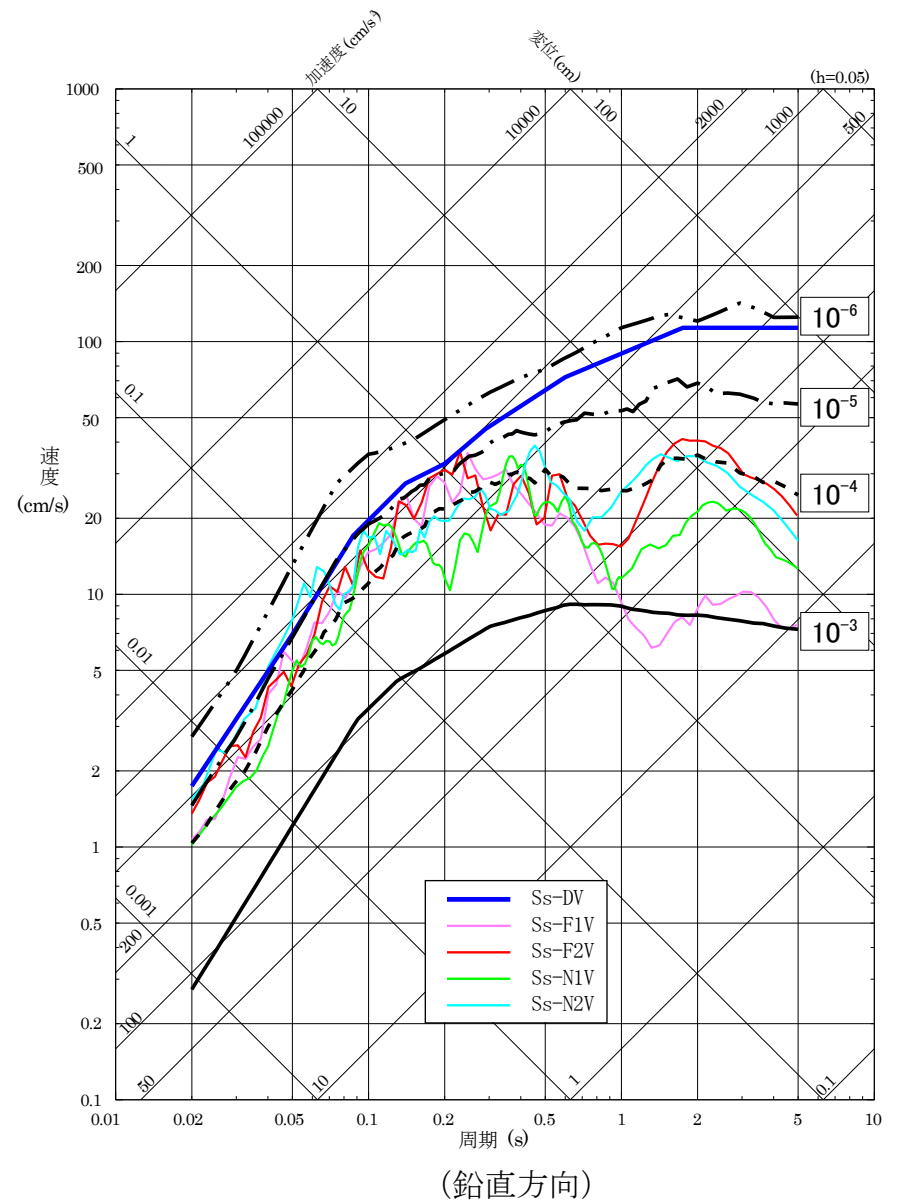
基準地震動 S_s の応答スペクトル及び解放基盤表面における地震動の一様ハザードスペクトルの比較
