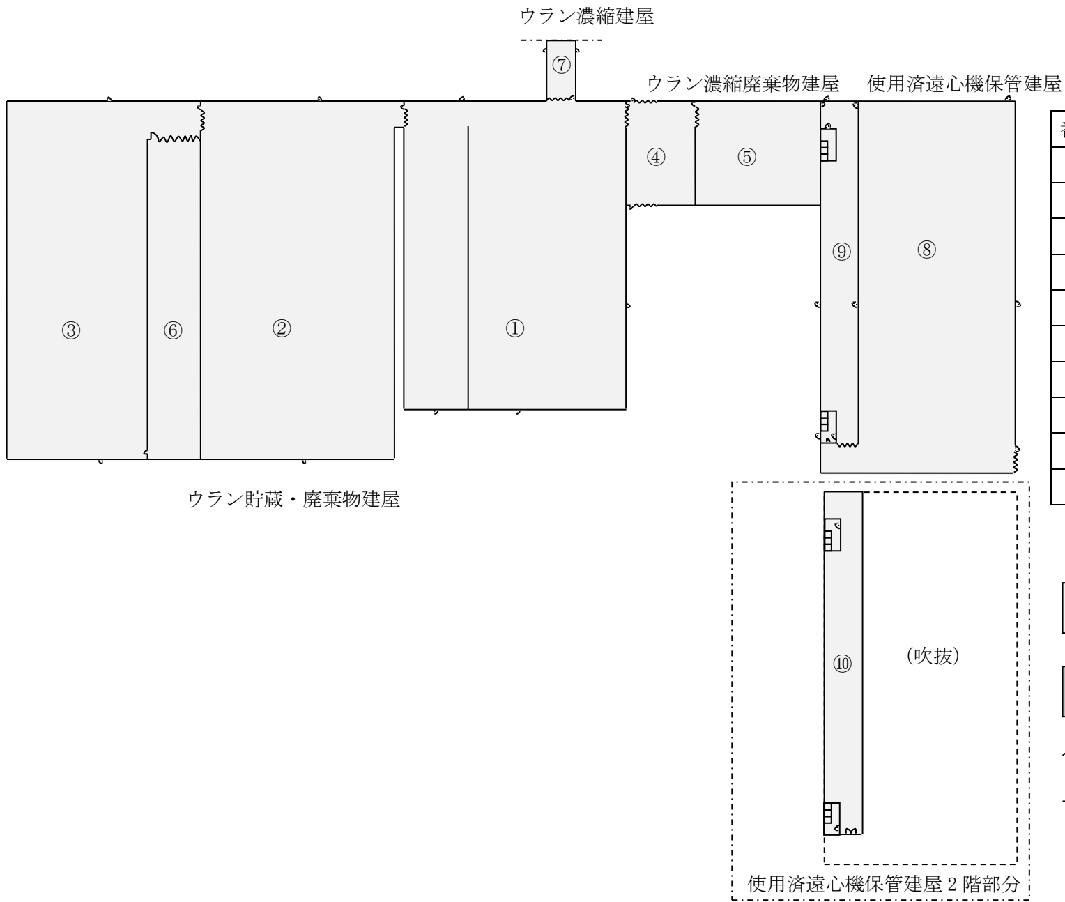
別図2 (3/3) ウラン貯蔵・廃棄物建屋、ウラン濃縮廃棄物建屋及び使用済遠心機保管建屋 管理区域図 (第45、49、54、55条関係)
