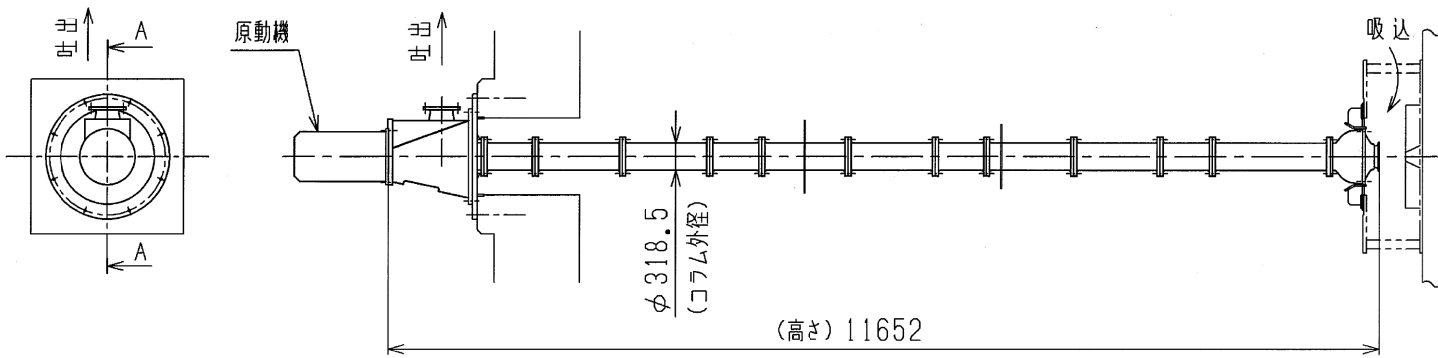
外形図
