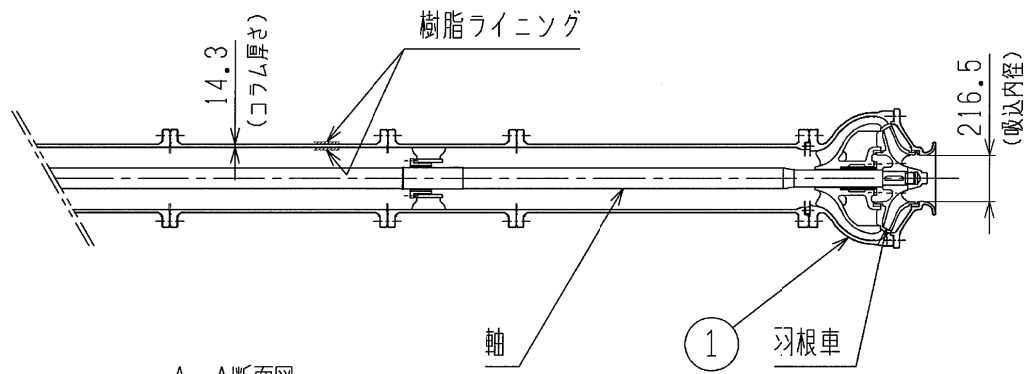
A~A断面図
