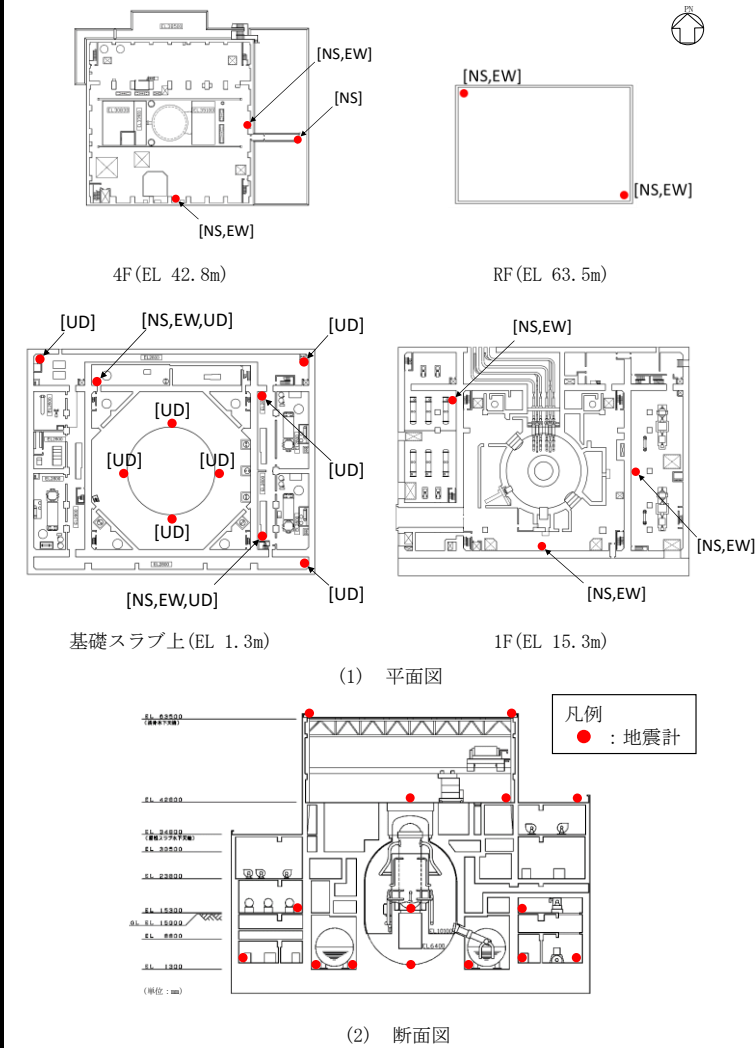
図3-1 地震計配置図 (原子炉建物)
