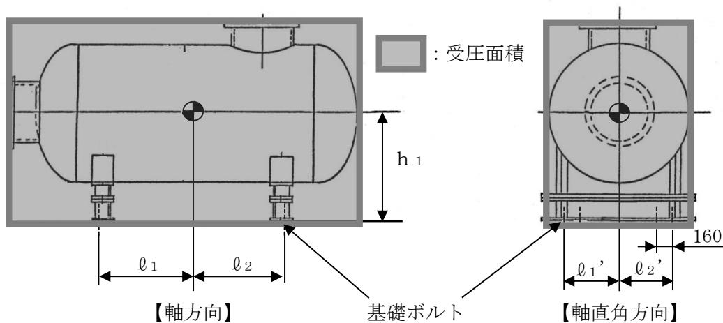
図3-1 排気消音器の基礎ボルト位置図
