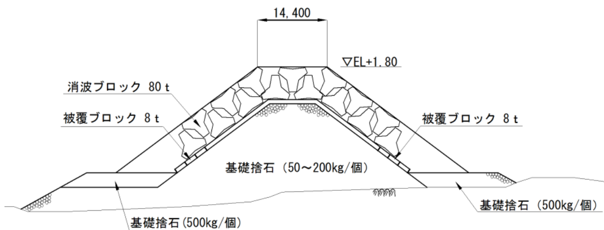
図4 東防波堤の構造概要
