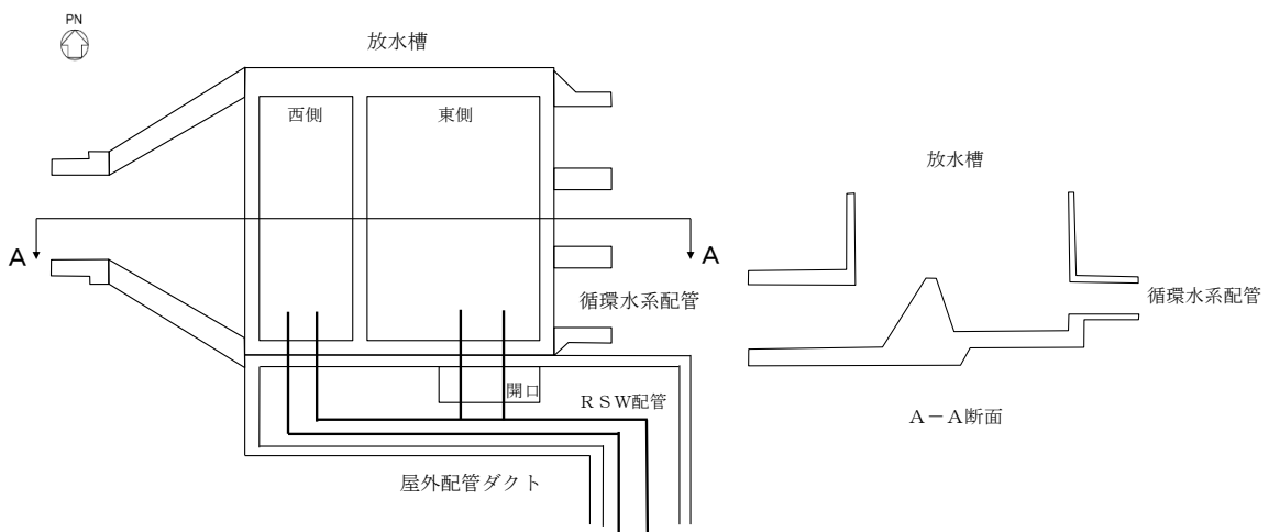
図3 放水槽の概略構造図
