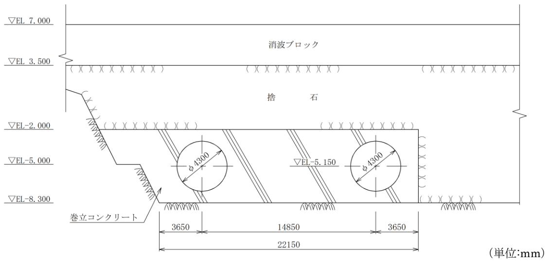
図8 取水管縦断方向断面図
