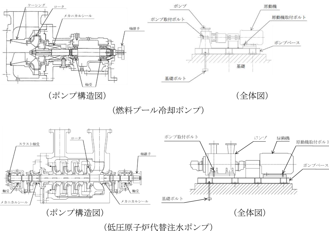
別紙 2-1-1 図 横形ポンプの構造概要図
