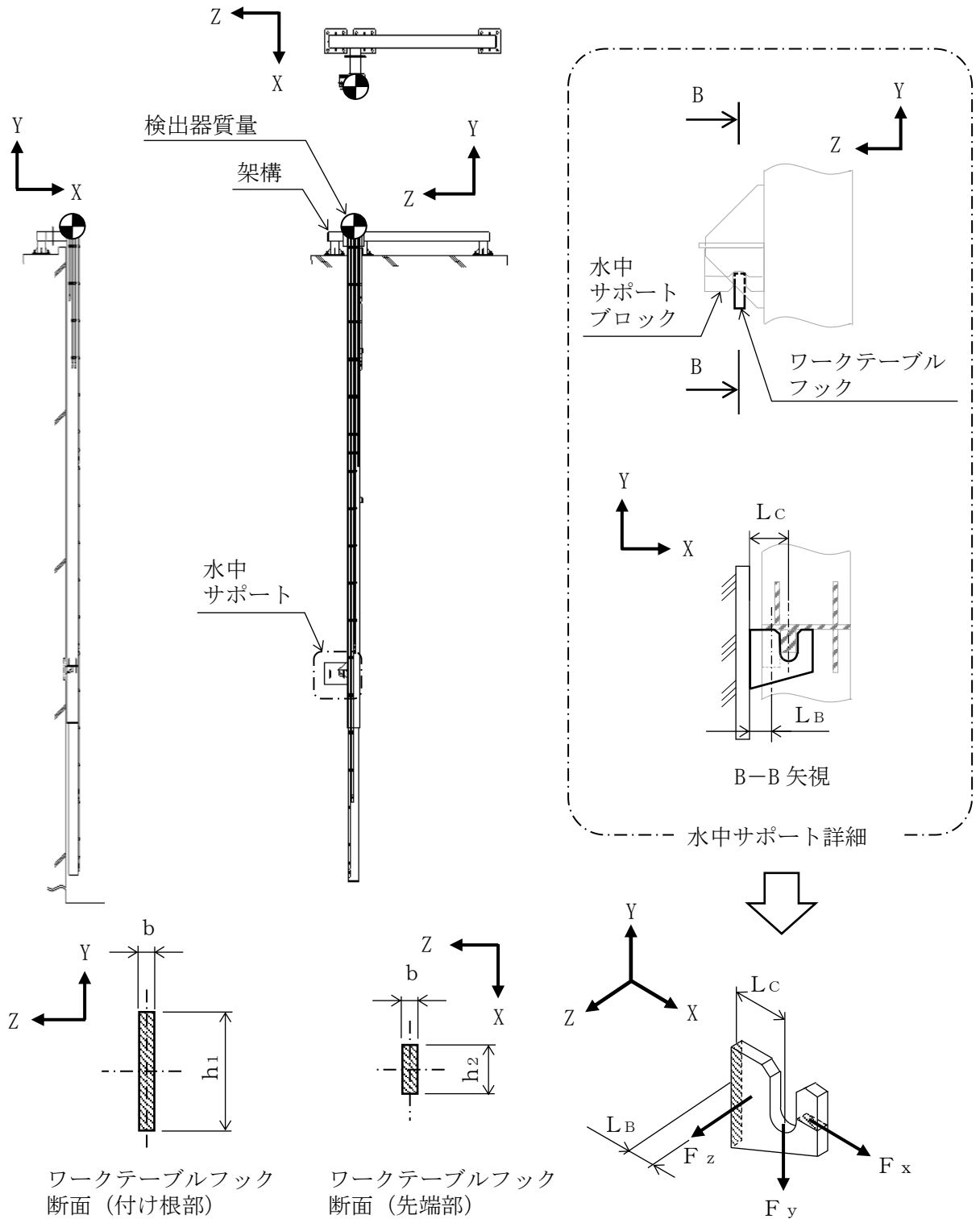
図5-2 構造概要 (ワークテーブルフック)
