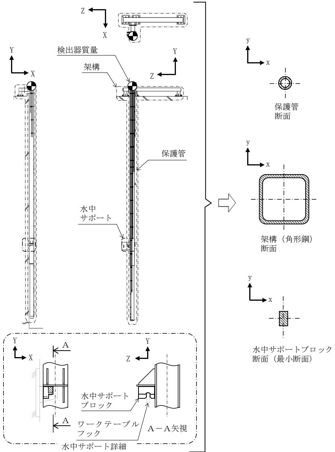
図 5-2 構造概要 (架構)
