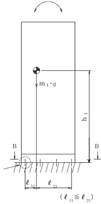
側面 (短辺方向) 転倒方向
