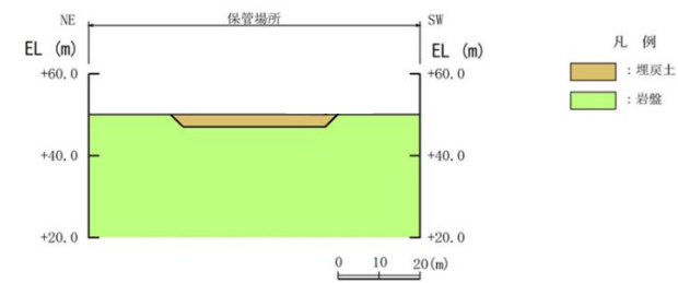
図 2-6 液状化及び揺すり込みによる不等沈下・傾斜に対する影響評価断面位置及び断面図 (第 1 保管エリア)
