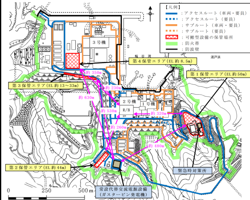
保管場所と原子炉建物及び常設代替交流電源設備との離隔距離
