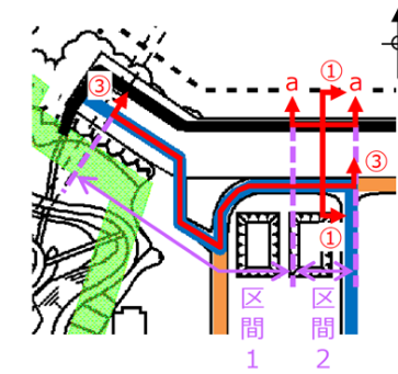
3号機北西側アクセスルート拡大図
