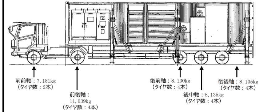
図 2-11 移動式代替熱交換設備の仕様
