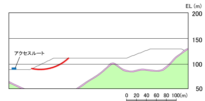
⑰-⑰' 断面
