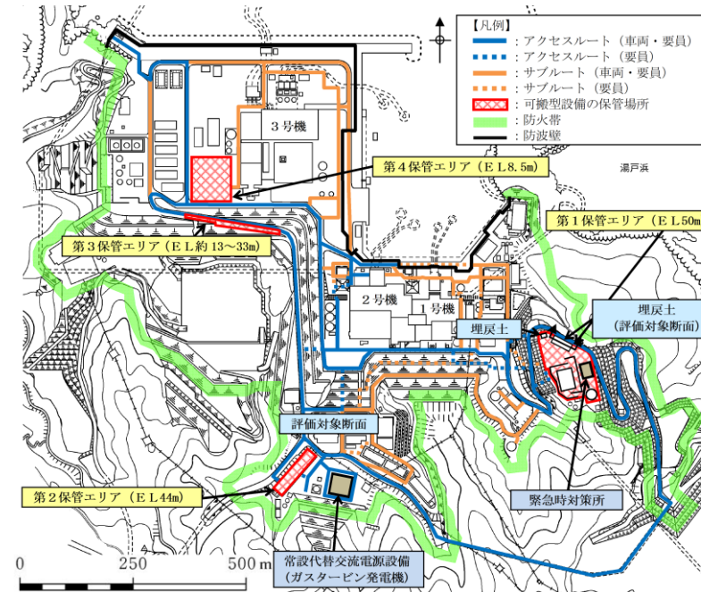
影響評価断面位置
