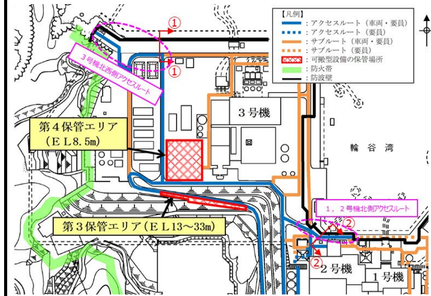
全体平面図
