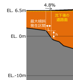
③-③断面
